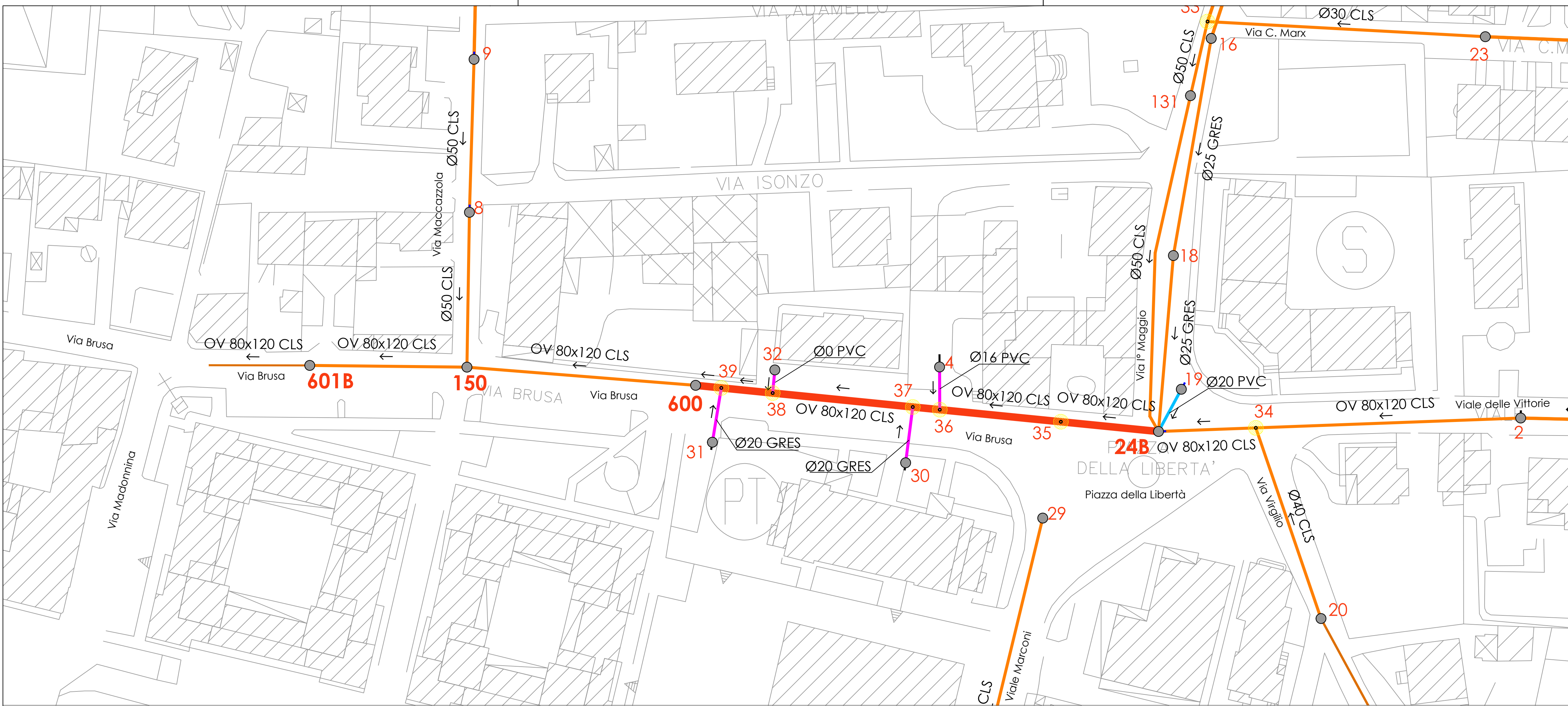
RETE FOGNARIA ESISTENTE, TRATTO INTERESSATO DALL'INTERVENTO, SCALA 1:200
