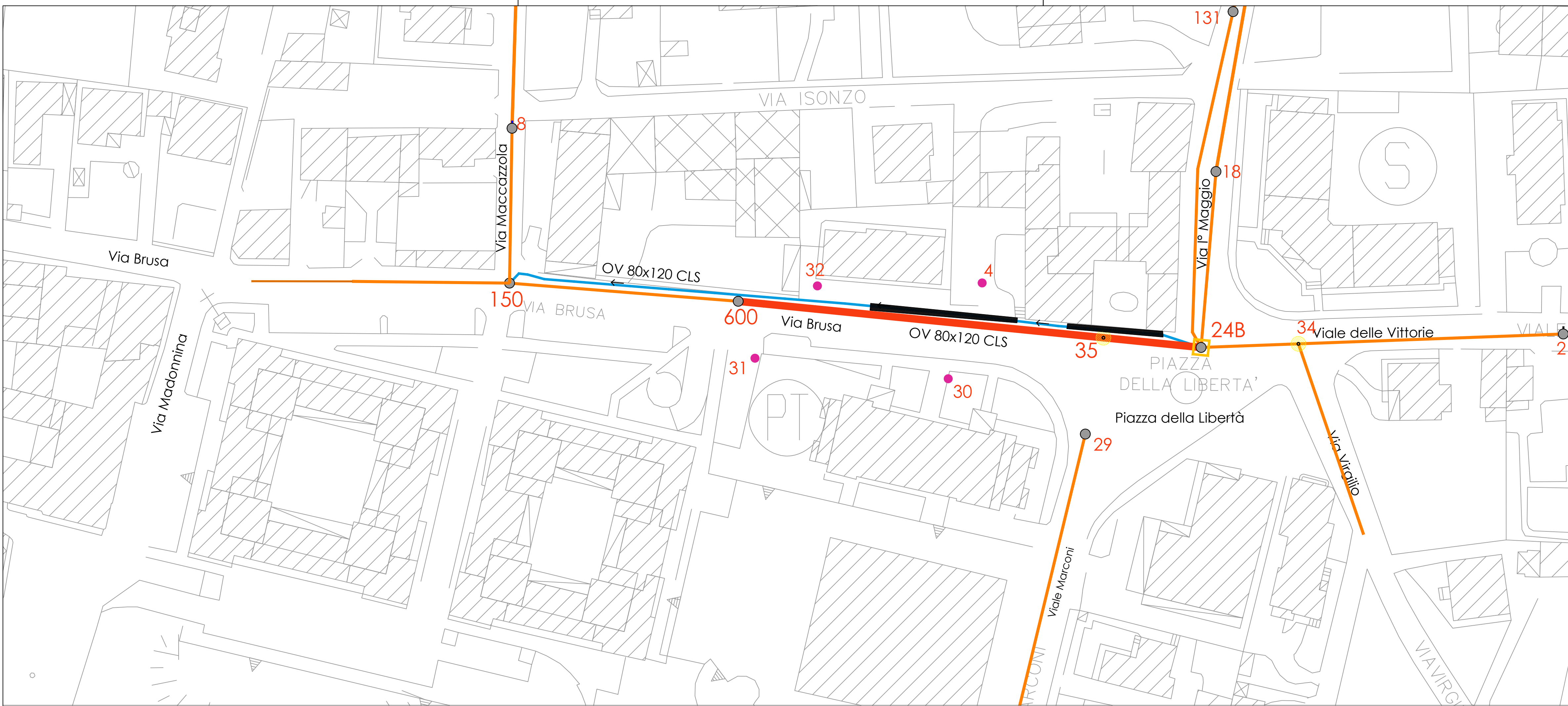
RETE FOGNARIA ESISTENTE_SCALA 1:500
