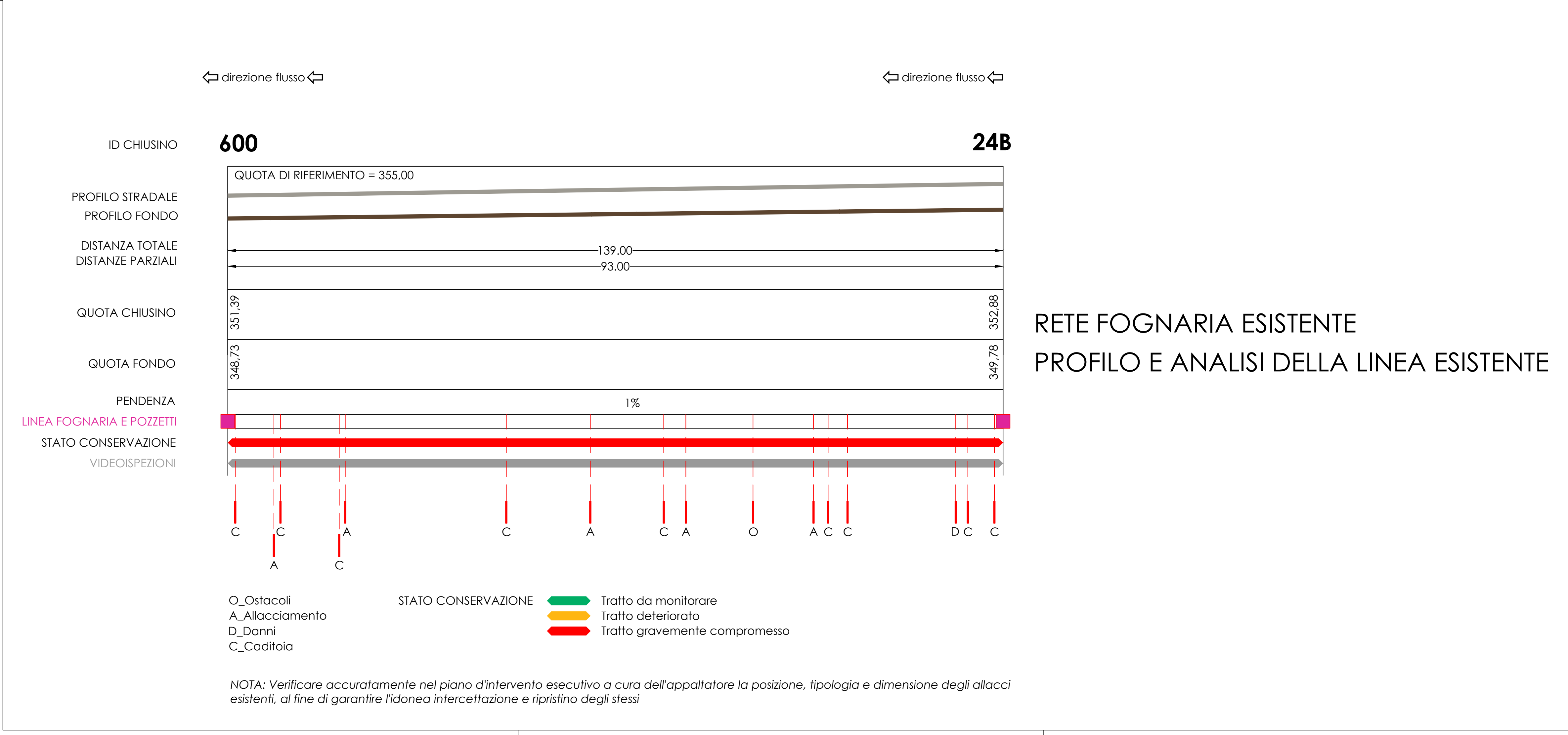
RETE FOGNARIA ESISTENTE_SCALA 1:500
