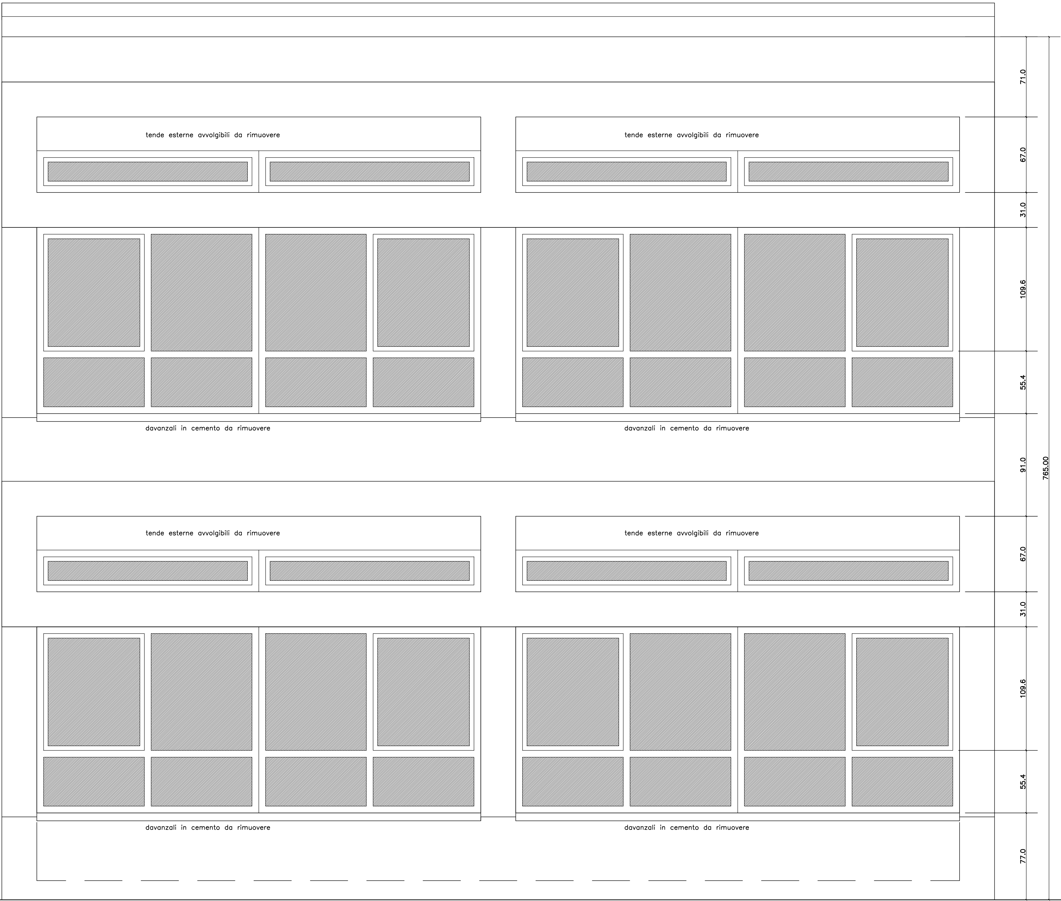
Prospetto esterno
