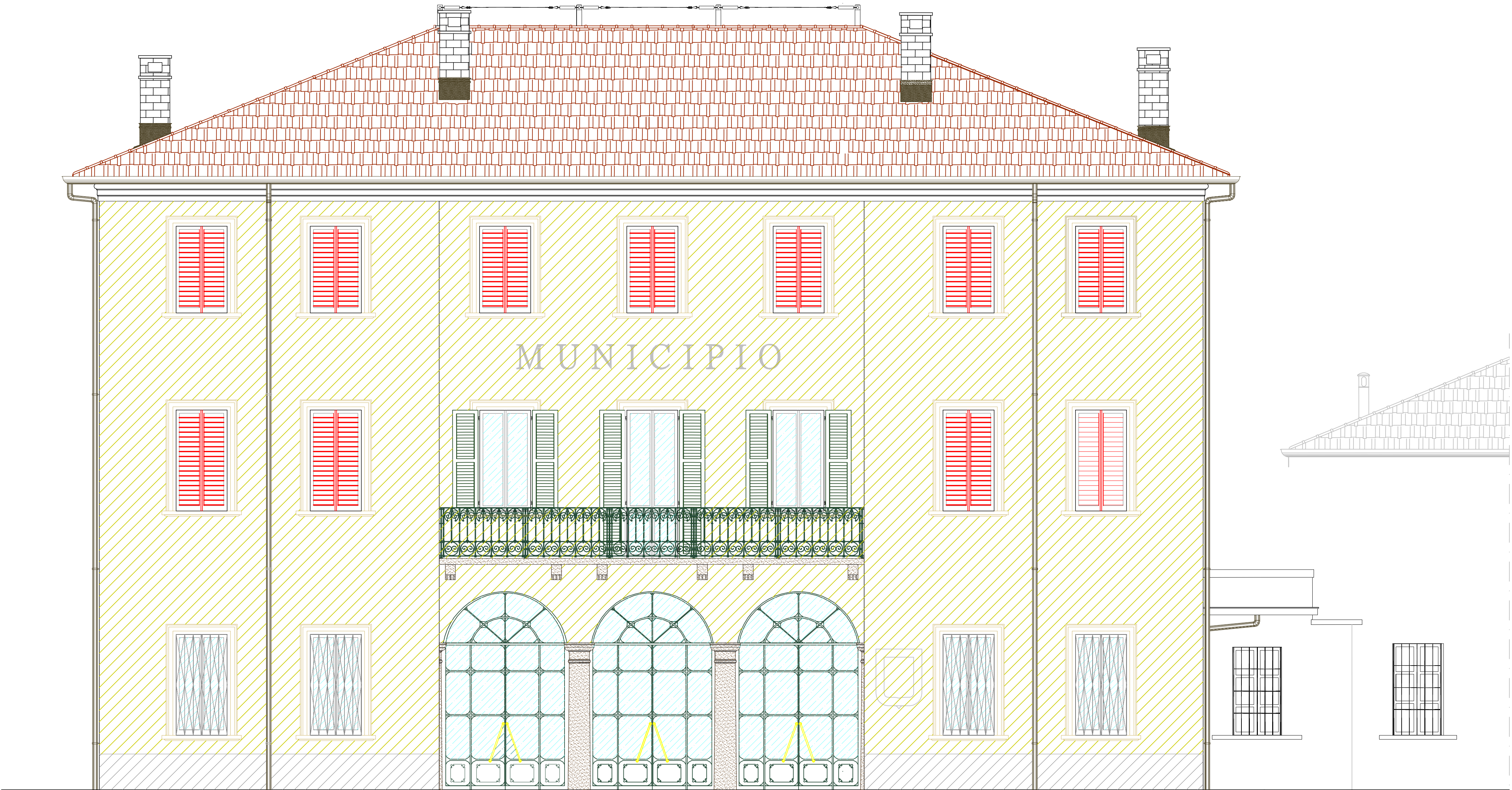
PROSPETTO SUD
