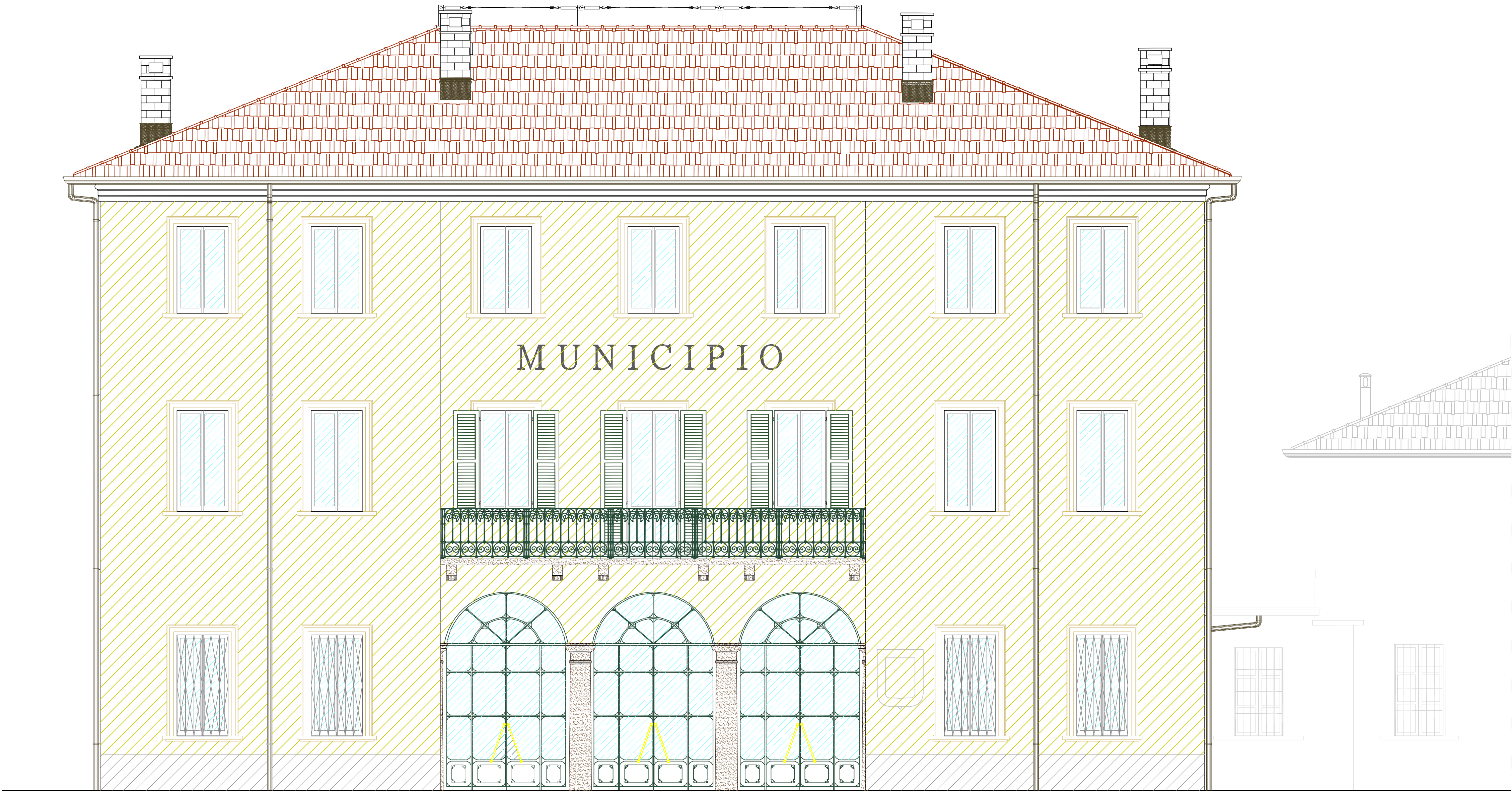
PROSPETTO SUD
