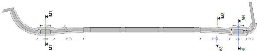
RECINZIONE PIANTA CARPENTERIE Scala 1:100
