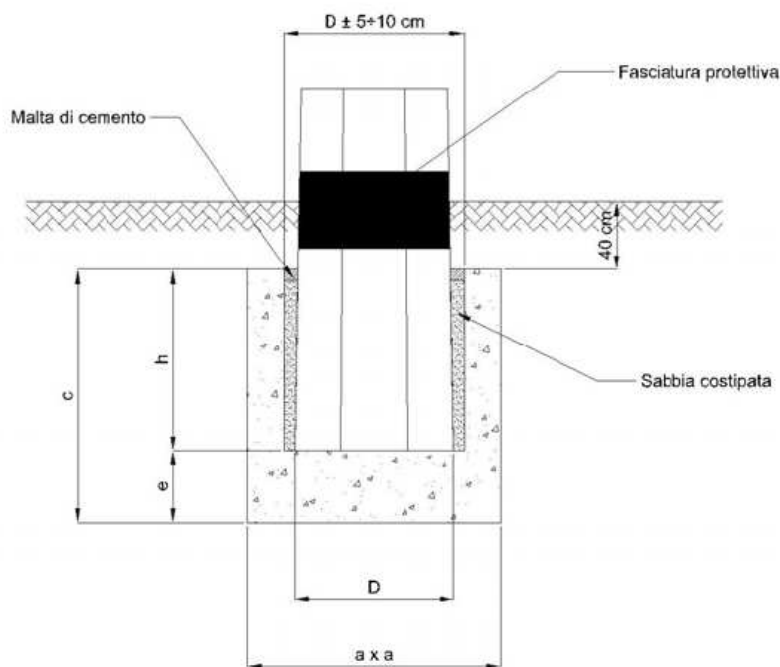
Fig. 1 - Blocco interrato
