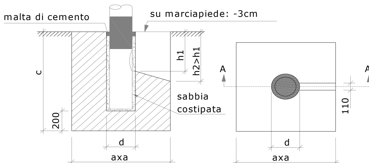
SEZIONE A-A
