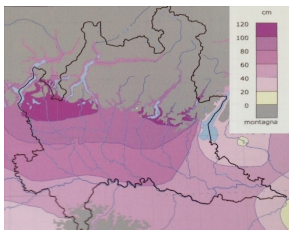
A sx.: Copertura del manto nevoso in Regione Lombardia in occasione della grande nevicata del 1985. A dx.: La neve al suolo a Milano in occasione della medesima nevicata – Immagine e foto tratte dall'“Atlante dei climi e microclimi della Lombardia” - Centro Meteorologico Lombardo (2011).
