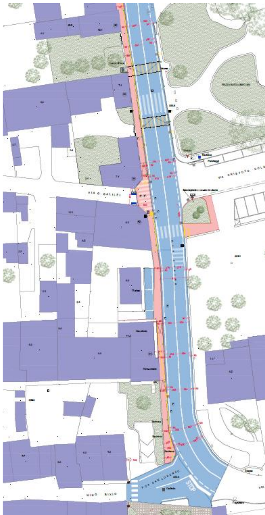
PLANIMETRIA INTERVENTO VIA RAVINA
