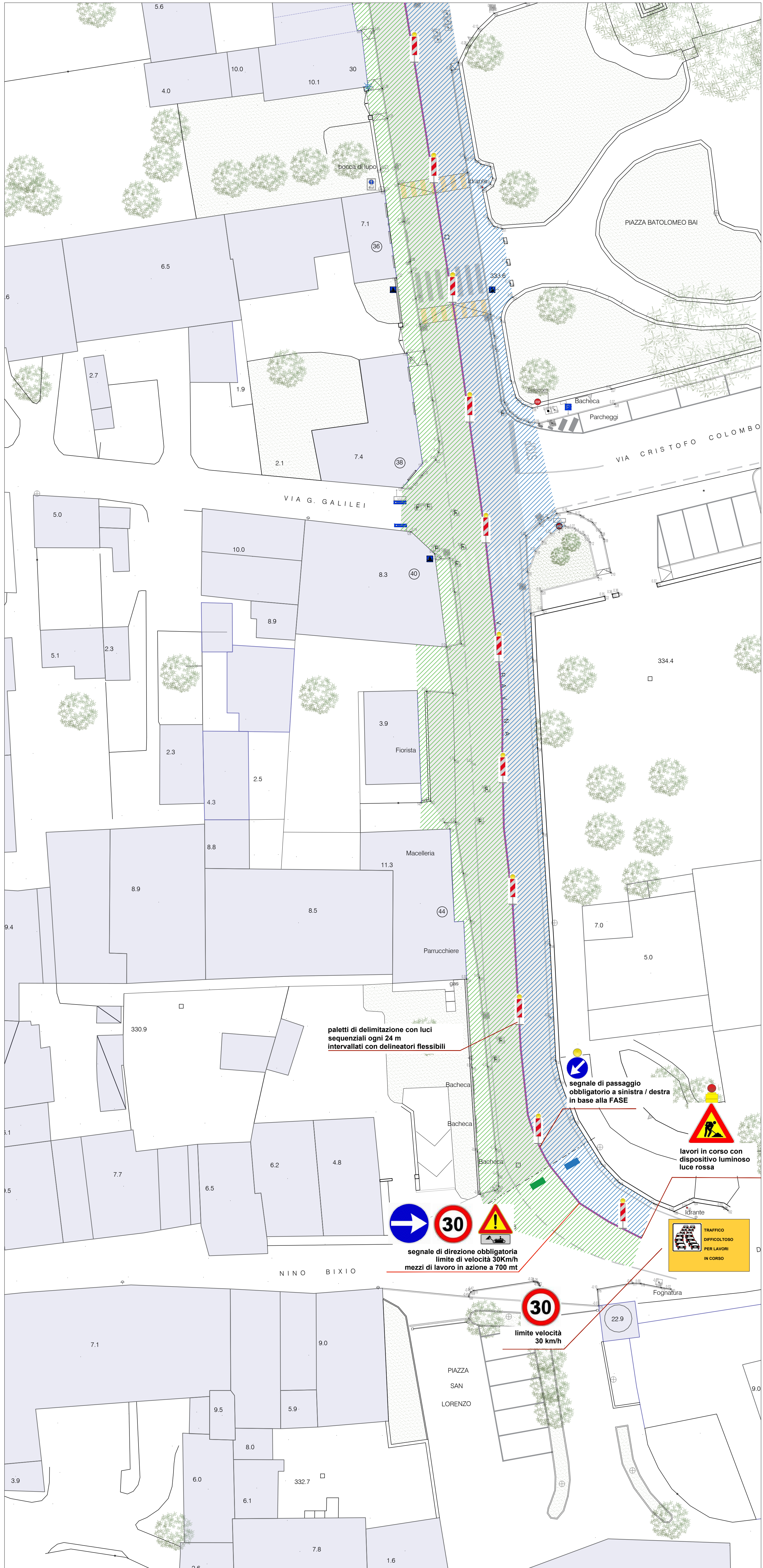
LAYOUT DI CANTIERE TRATTO 2
