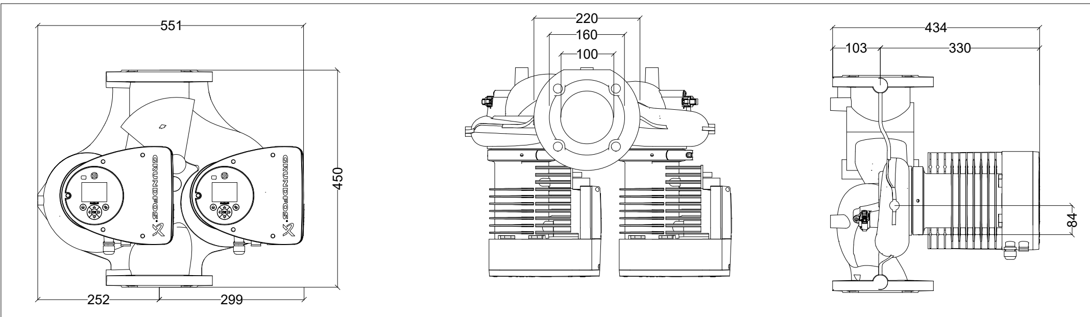
CIRCOLATORE MAGNA 3 D 100-120 F
