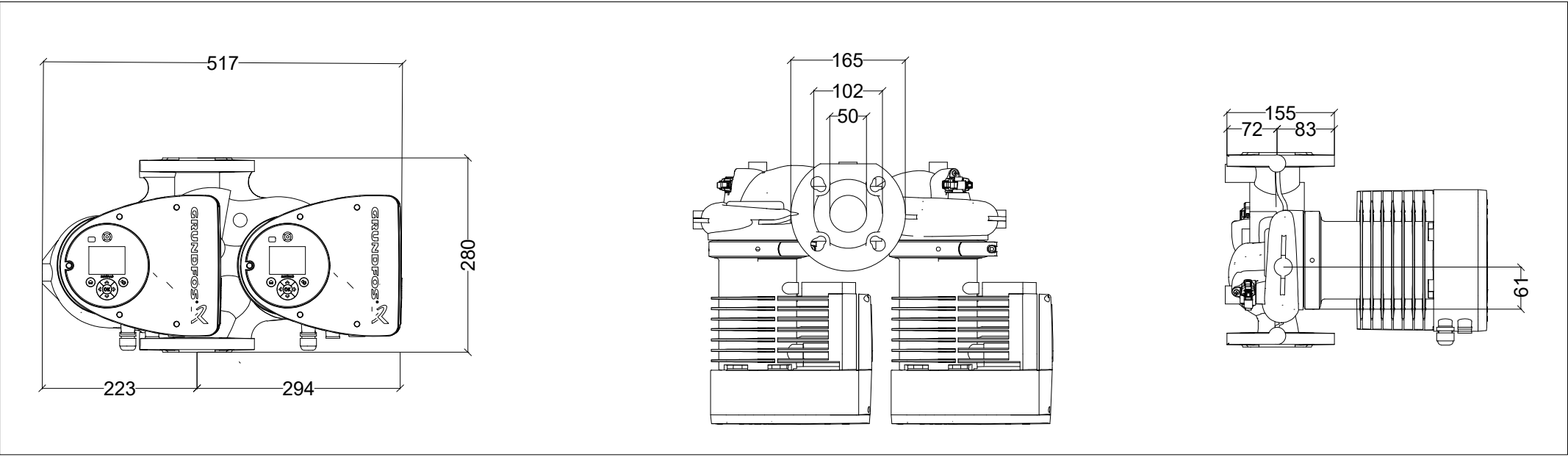
CIRCOLATORE MAGNA 3 D 65-80 F
