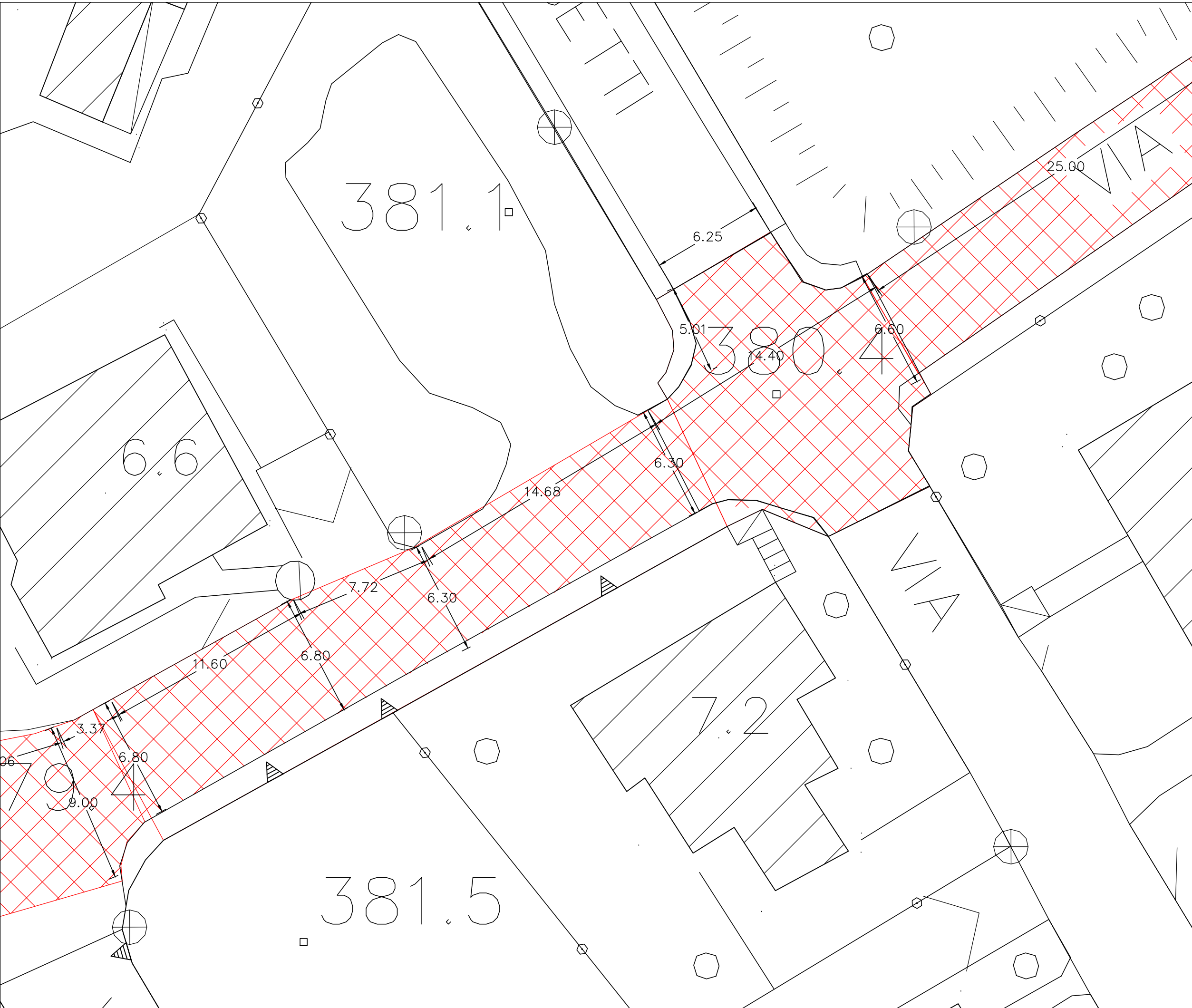
VIA MONTE CERVINO - ASFALTATURA E MODIFICA MARCIAPIEDE (B) - 1:200
