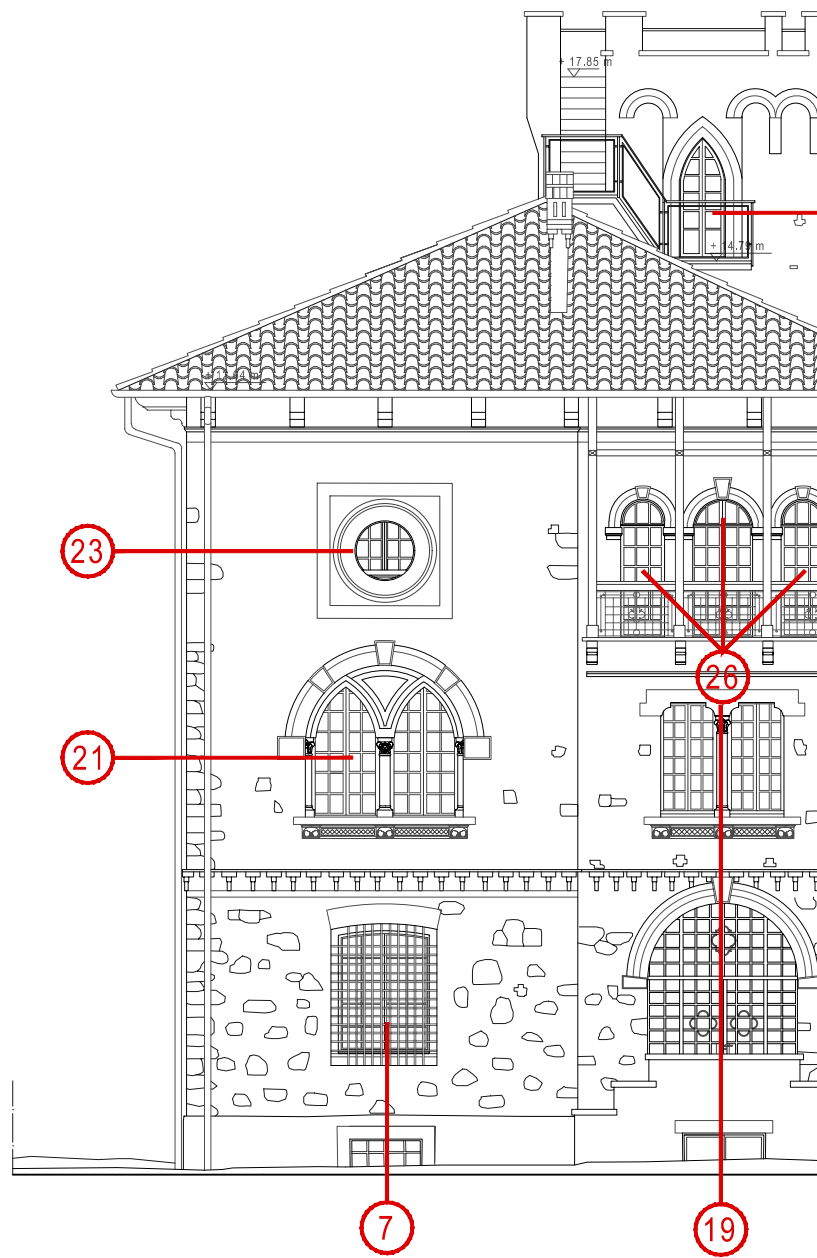
Prospetto OVEST
