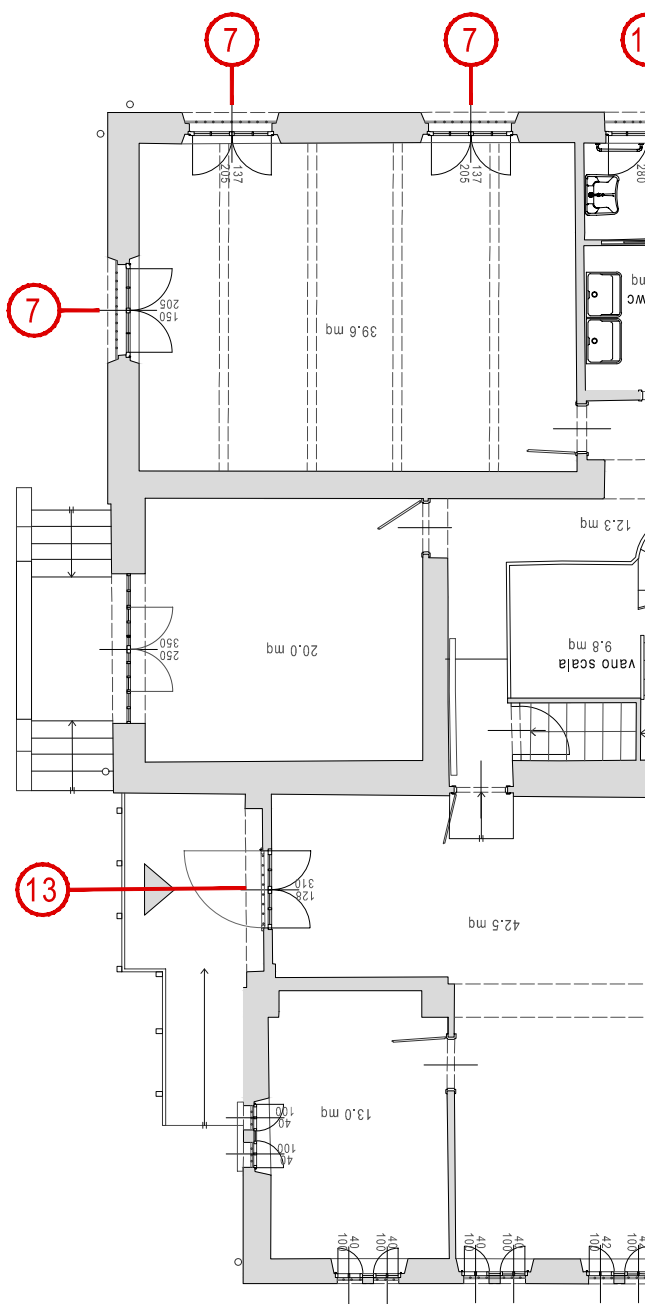
Planimetria Piano Rialzato
