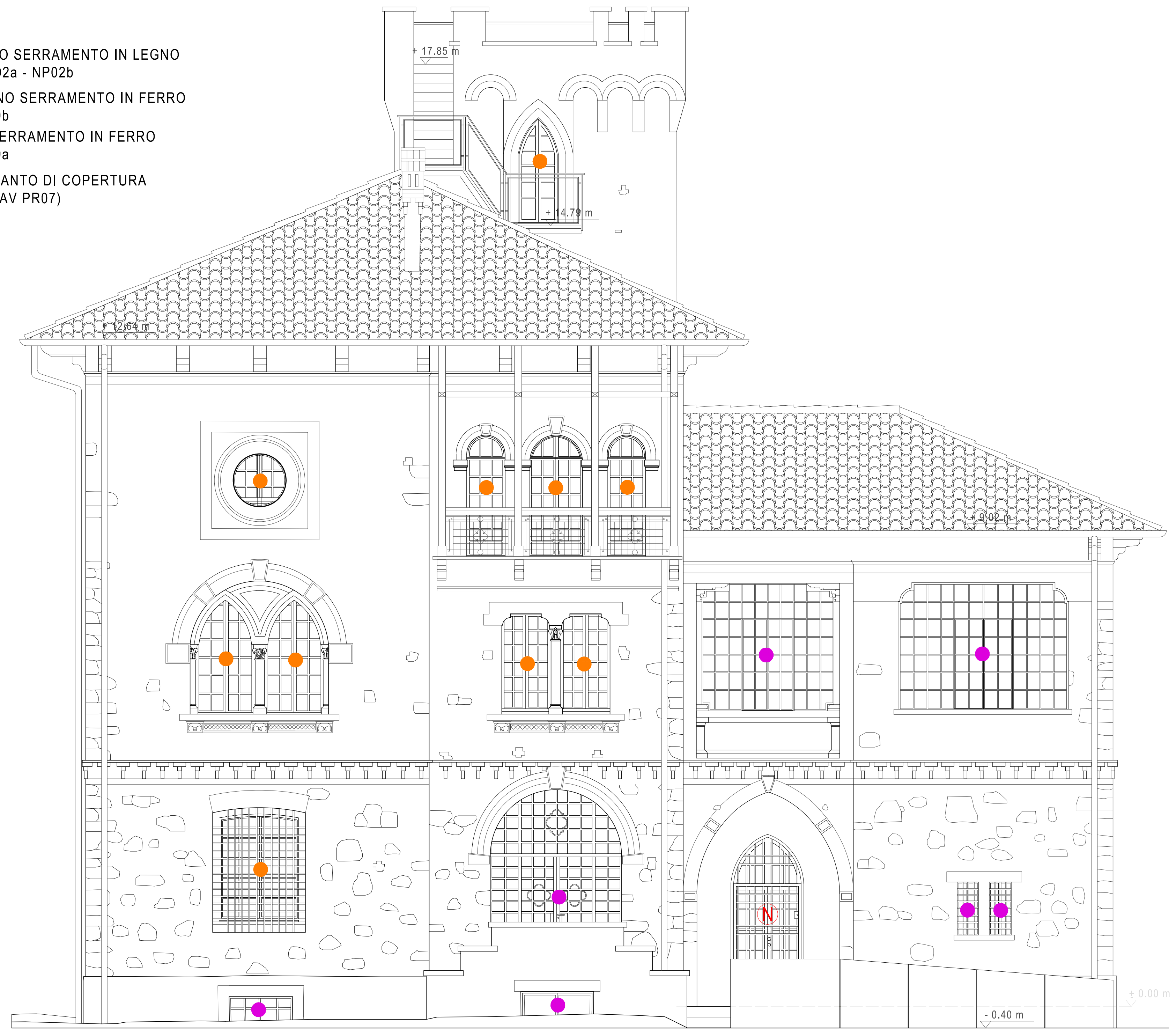
Prospetto OVEST
