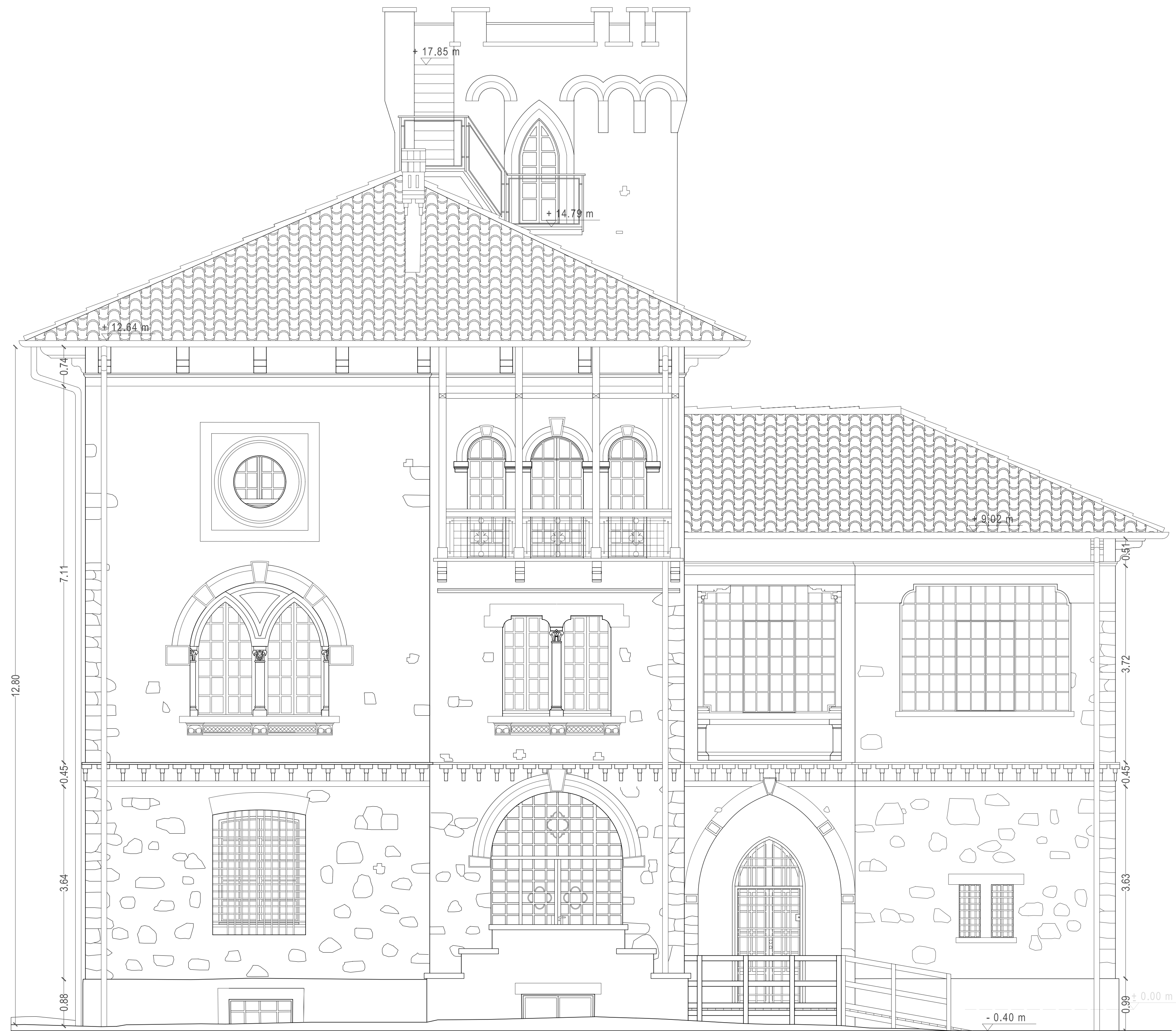
Prospetto OVEST
