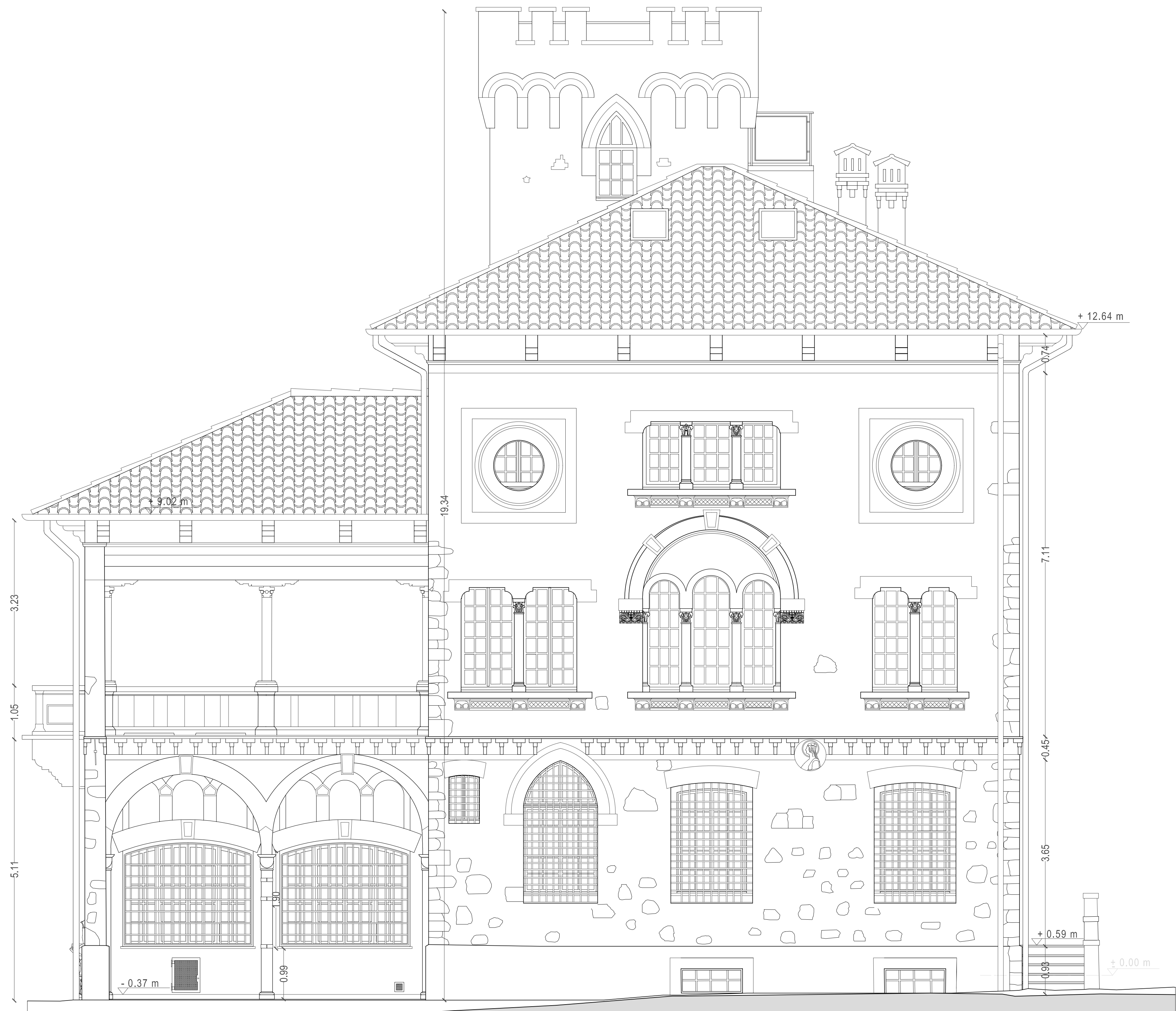
Prospetto NORD
