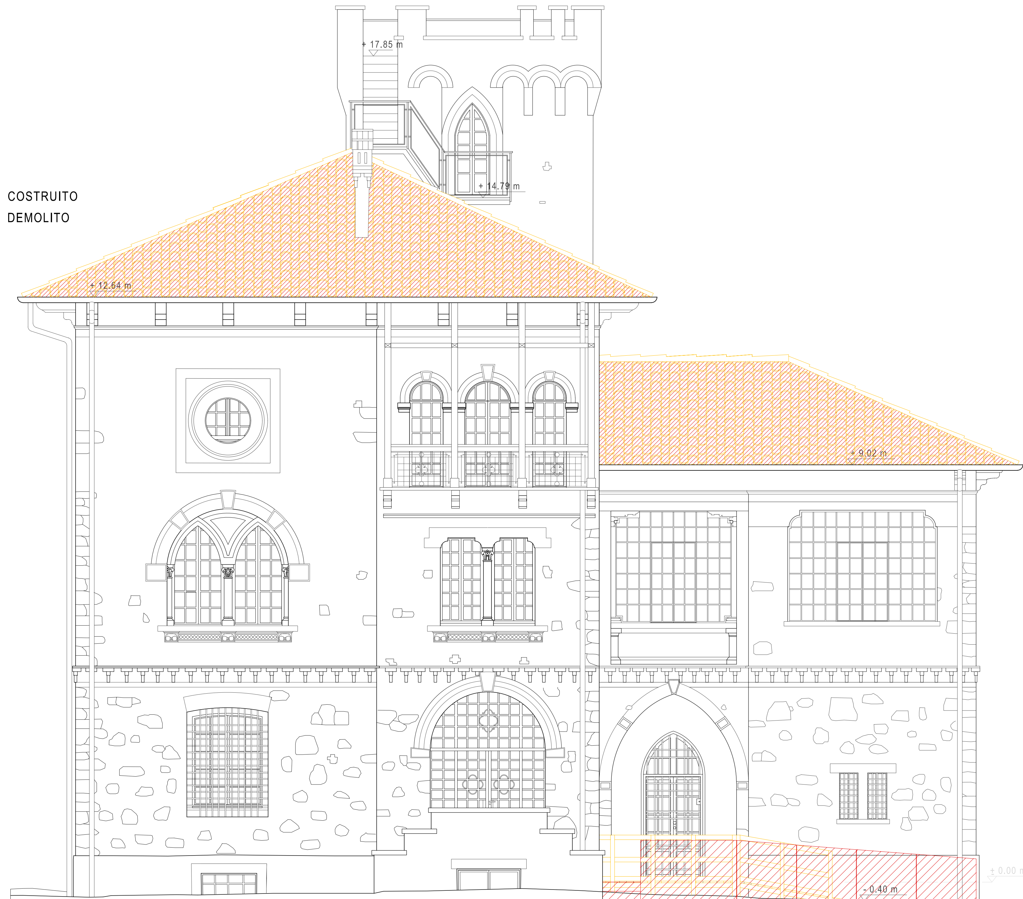
Prospetto OVEST
