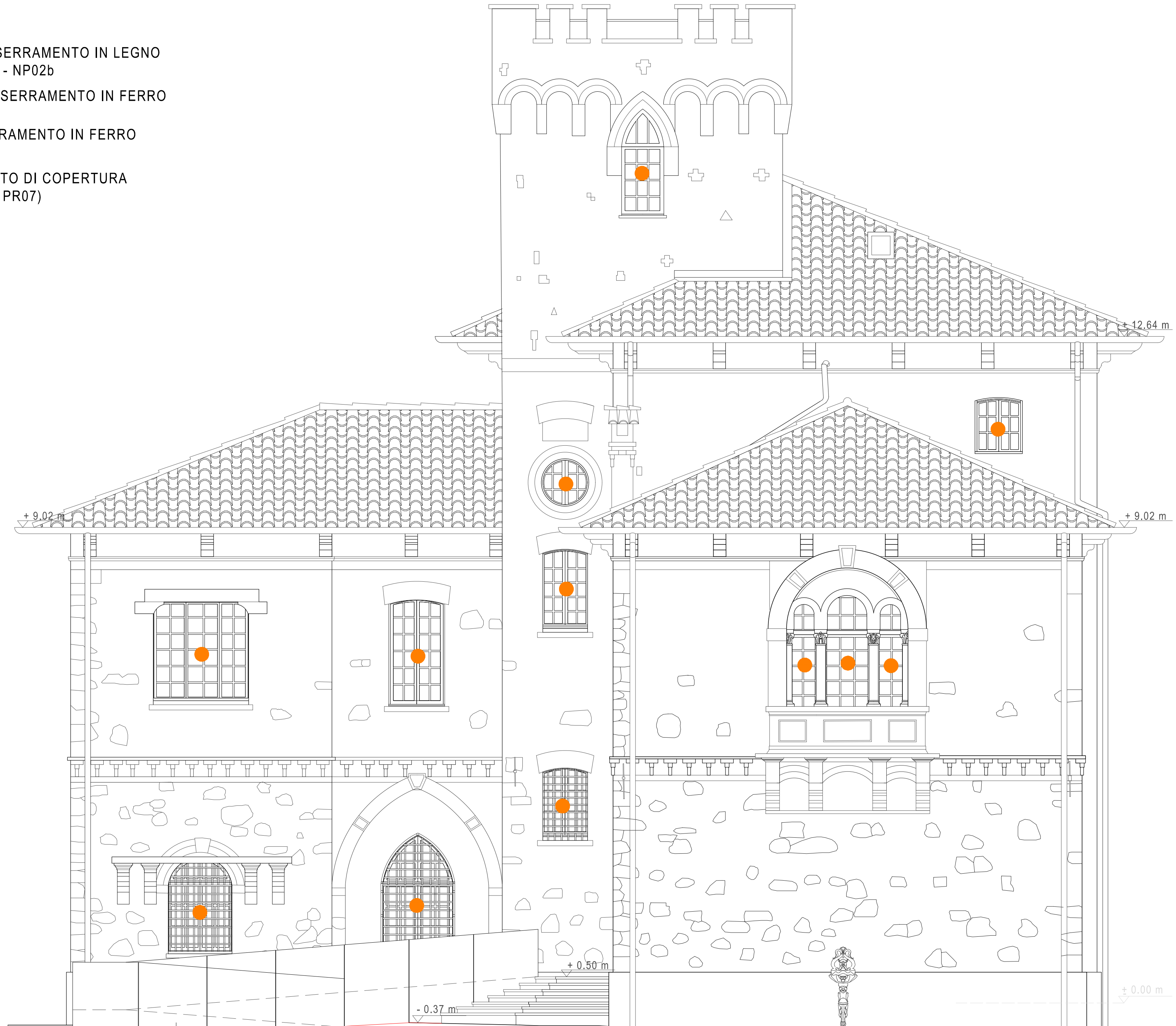
Prospetto EST
