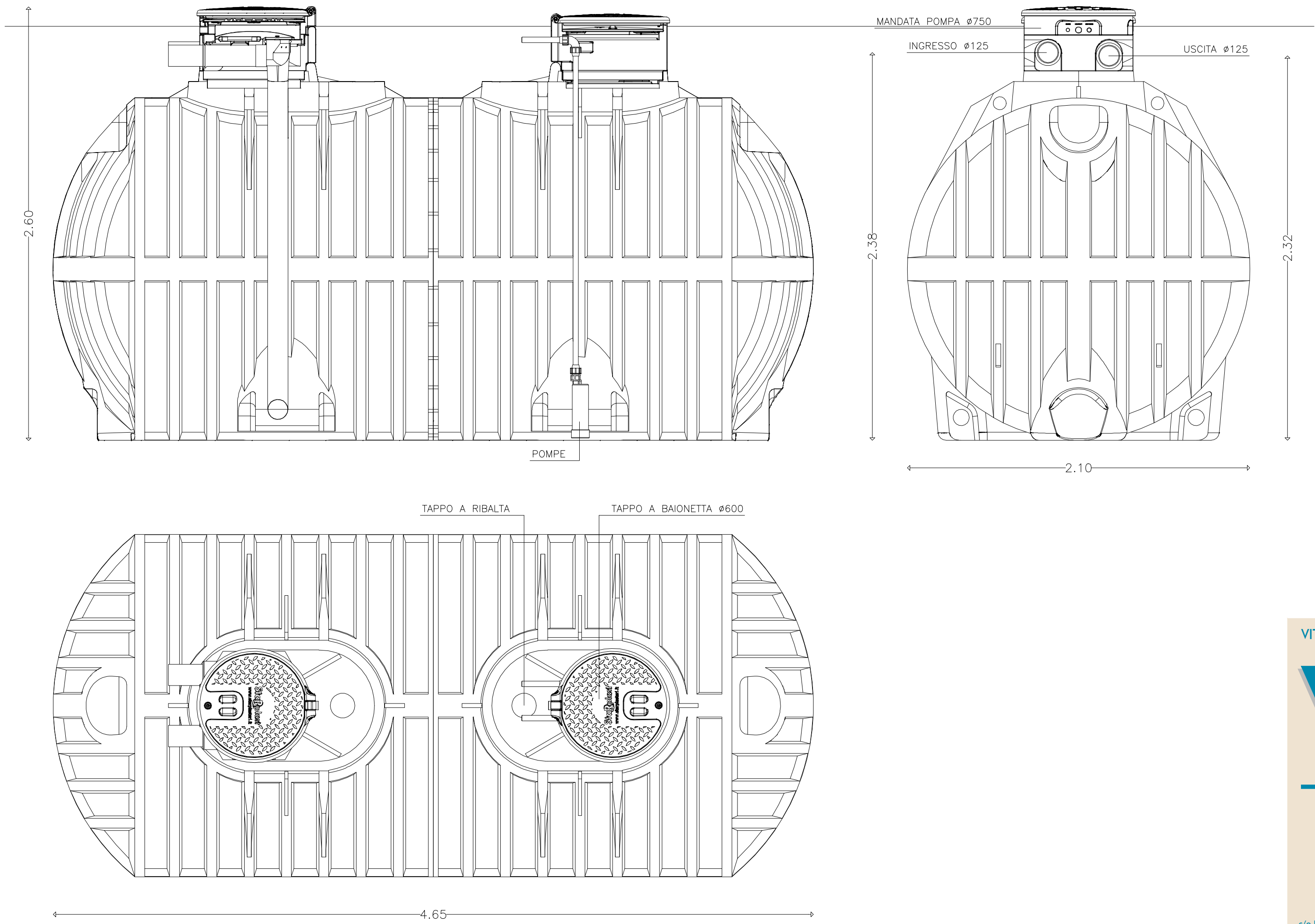
PARTICOLARE CISTERNA RISERVA IDRICA
