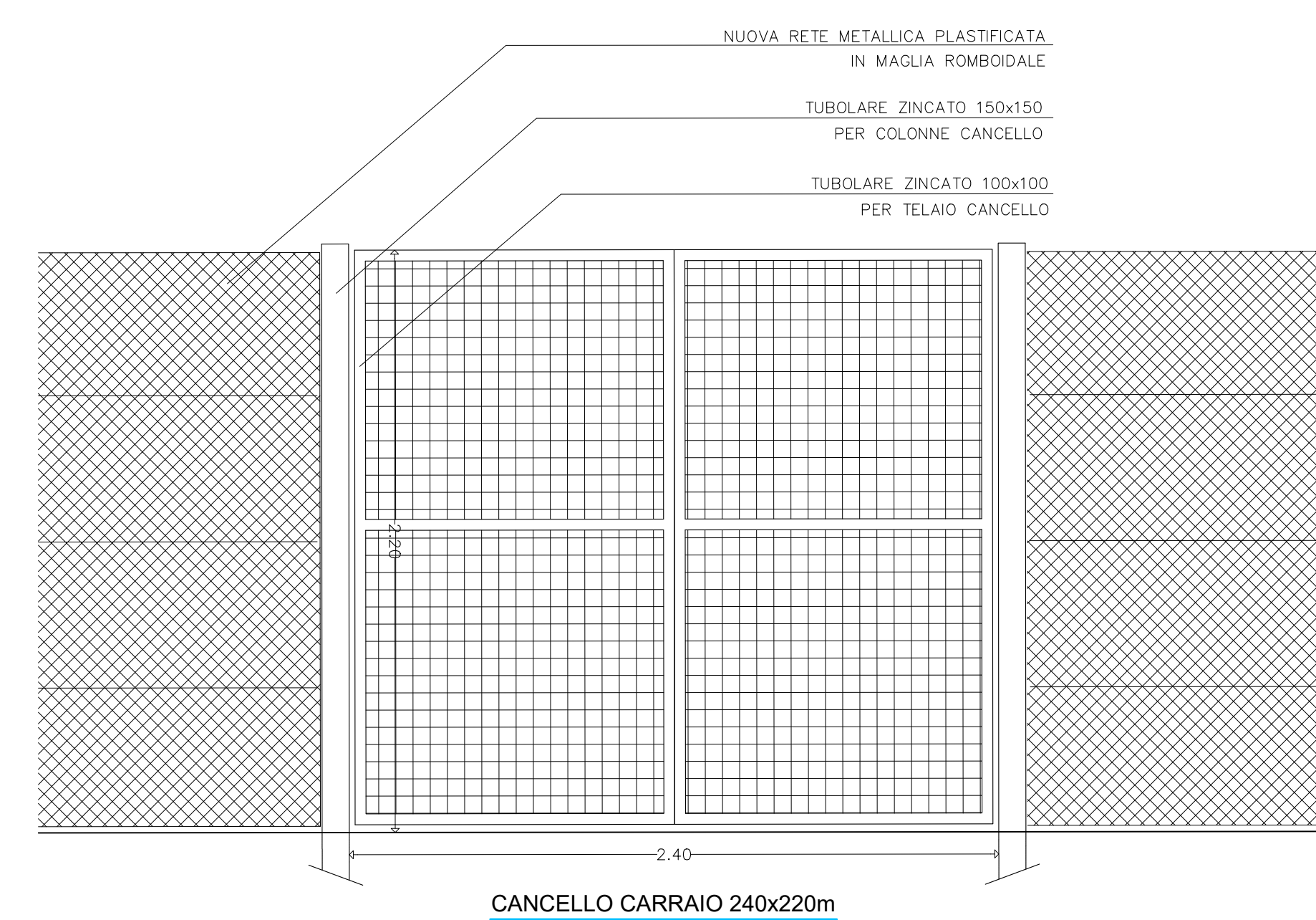
CANCELLO CARRAIO 240x220m
