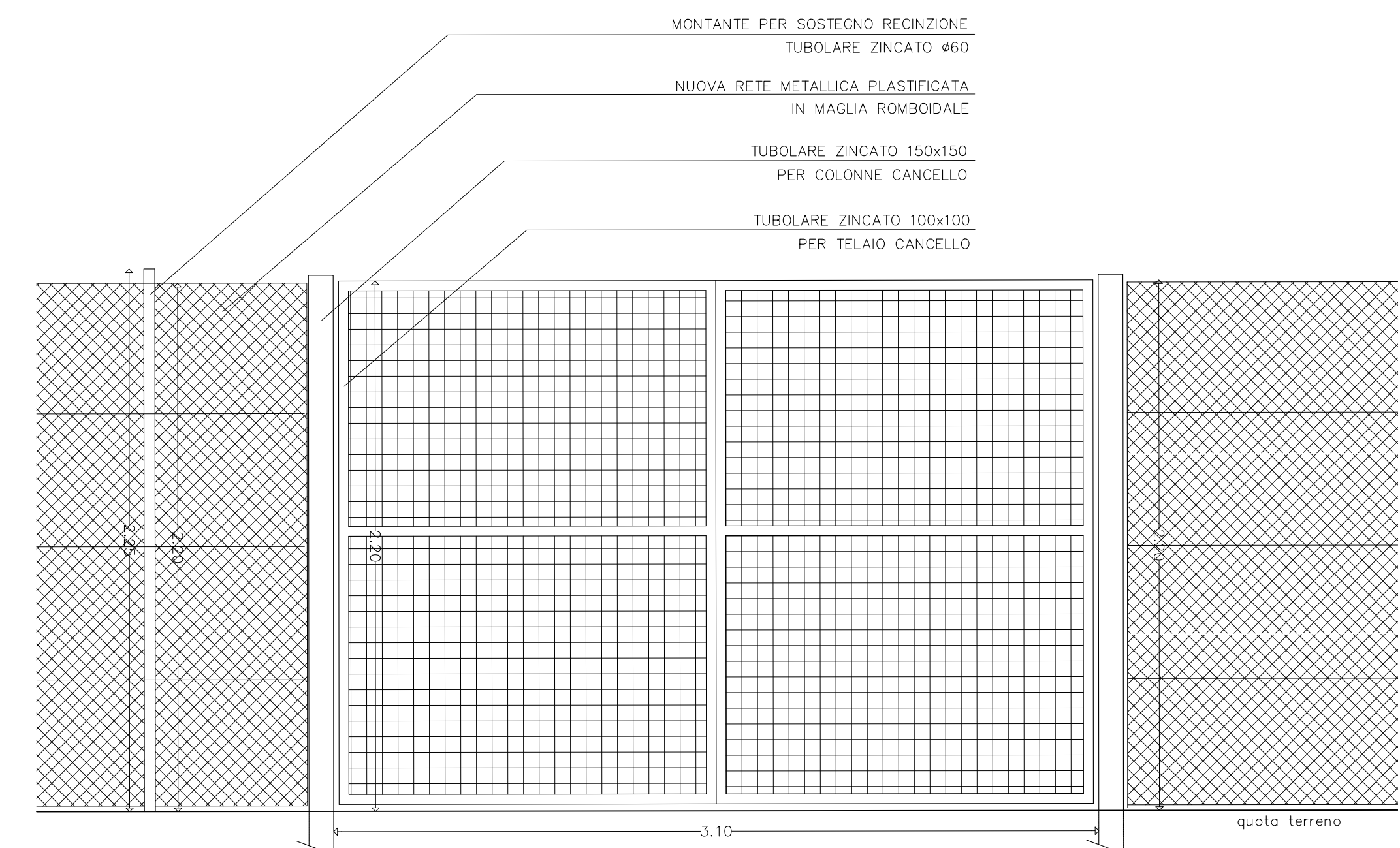
CANCELLO CARRAIO 310x220m
