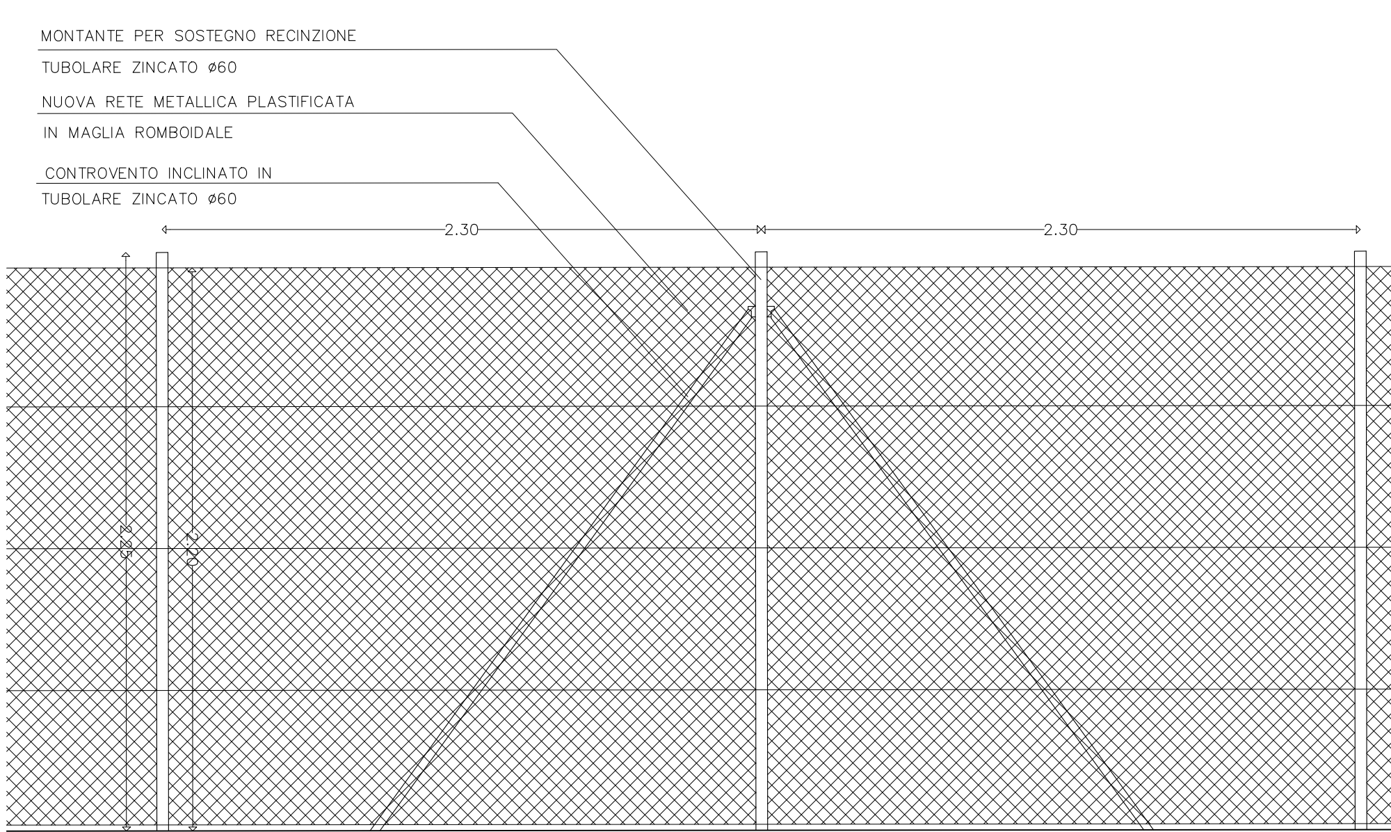
RECINZIONE SUI LATI MAGGIORI
