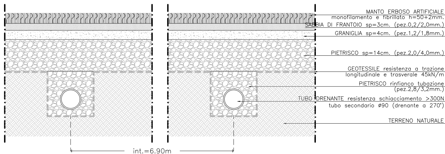
SOTTOFONDO DRENAGGIO INCLINATO CON INERTI SEZIONE A STRATI
