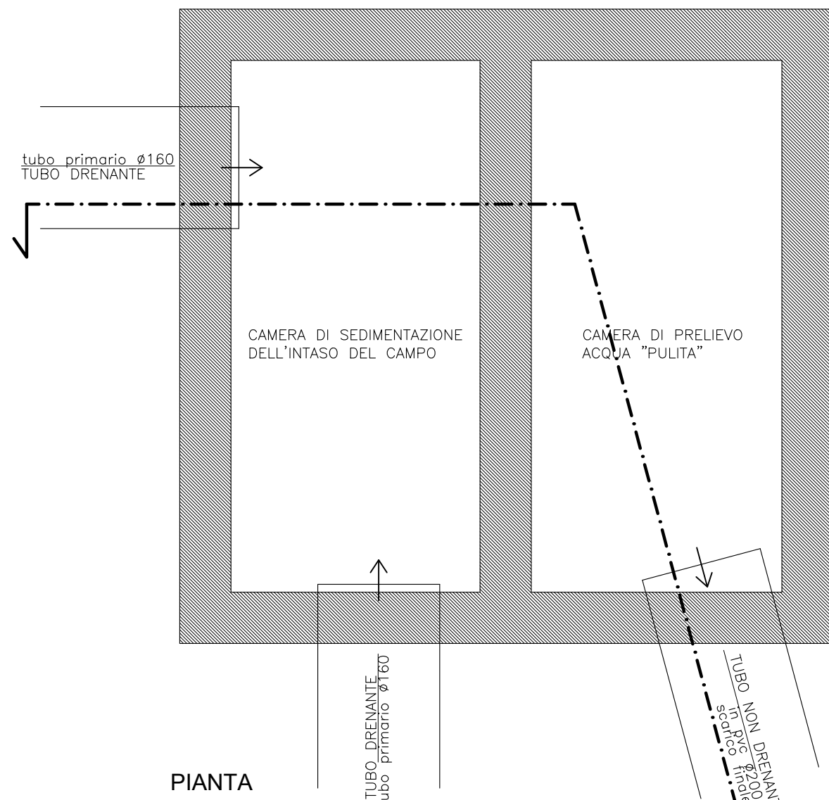
PARTICOLARE POZZETTO DI RACCOLTA 100x100 CM SIFONATO E DIFRAMMATO
