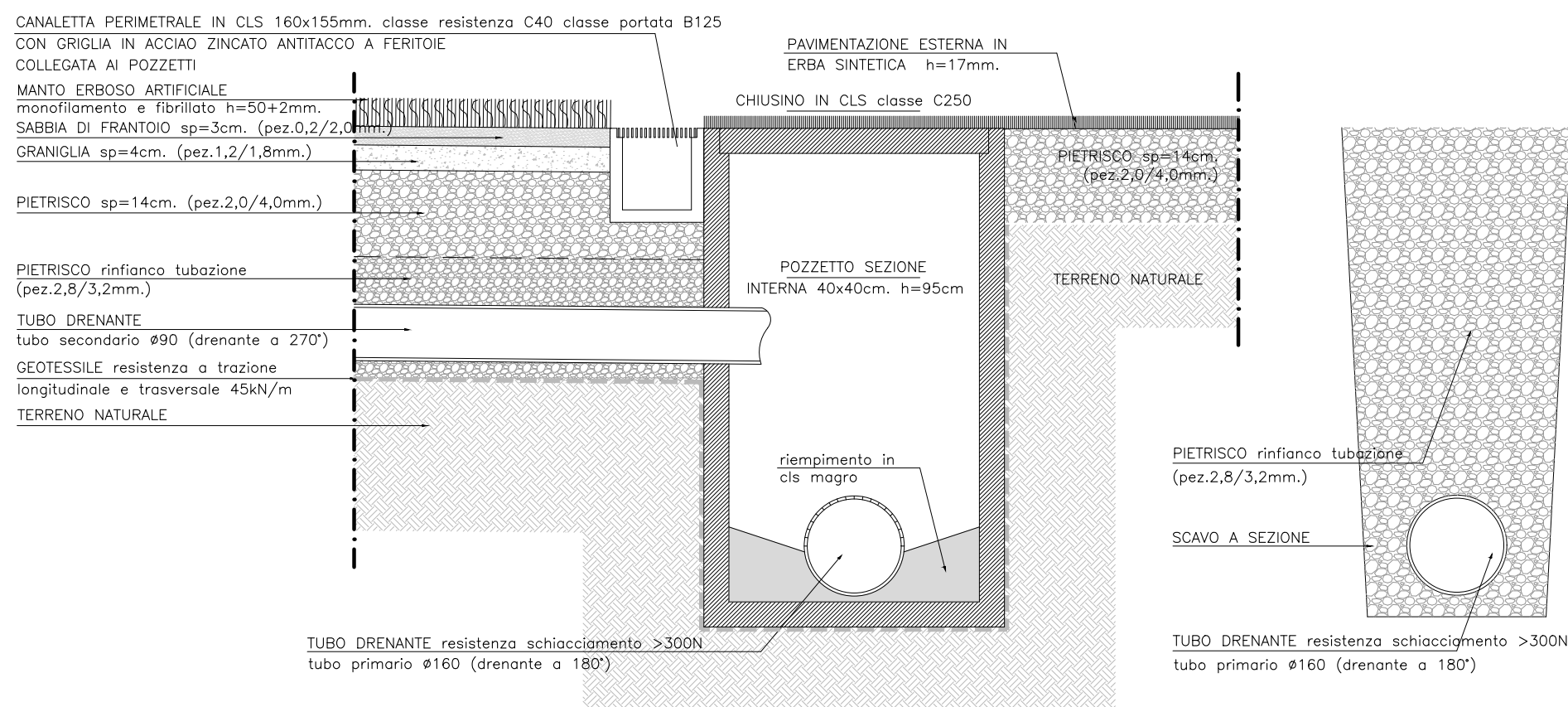
PARTICOLARE COSTRUTTIVO DRENAGGIO PERIMETRALE SEZIONE A STRATI
