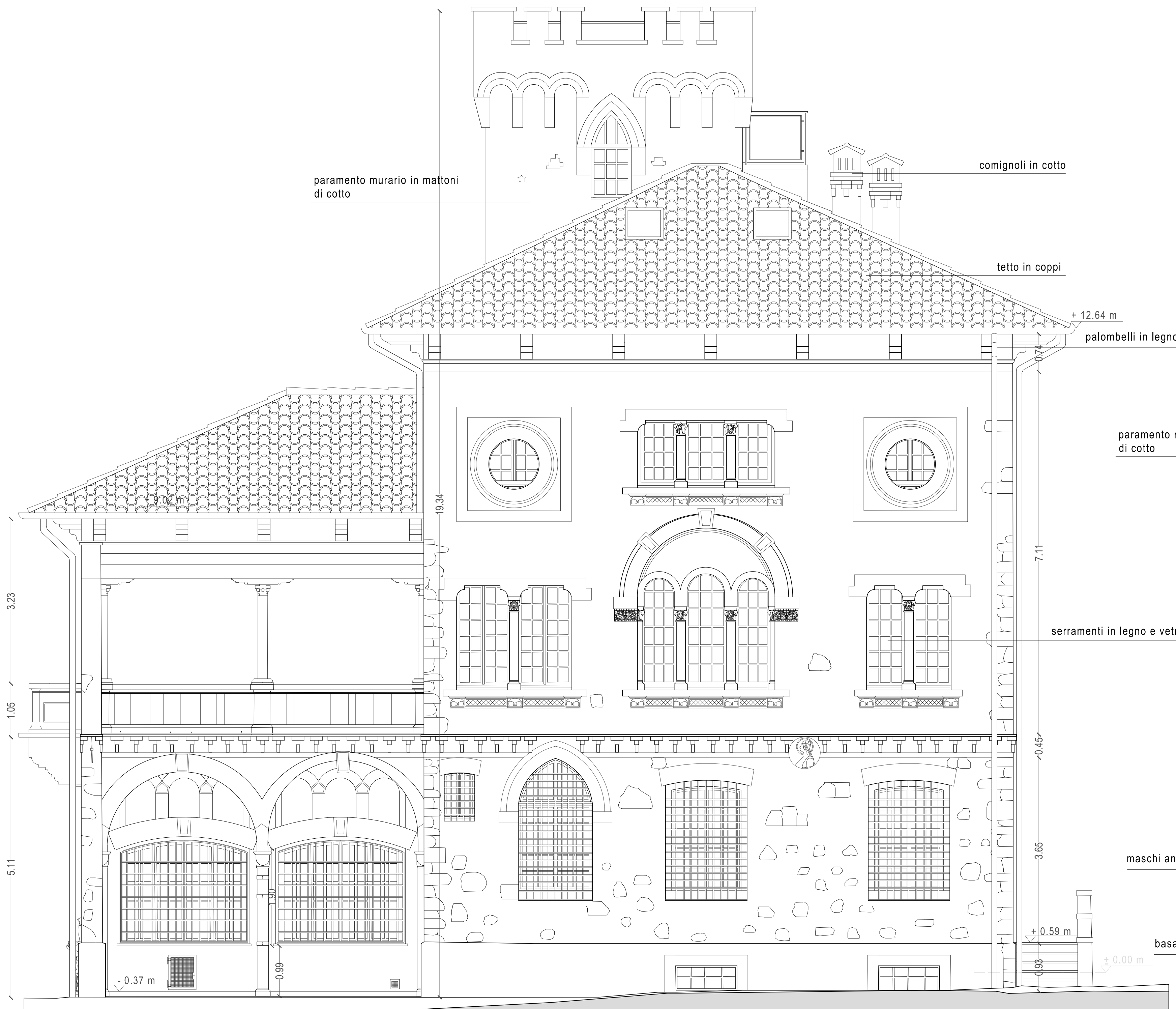
Prospetto NORD
