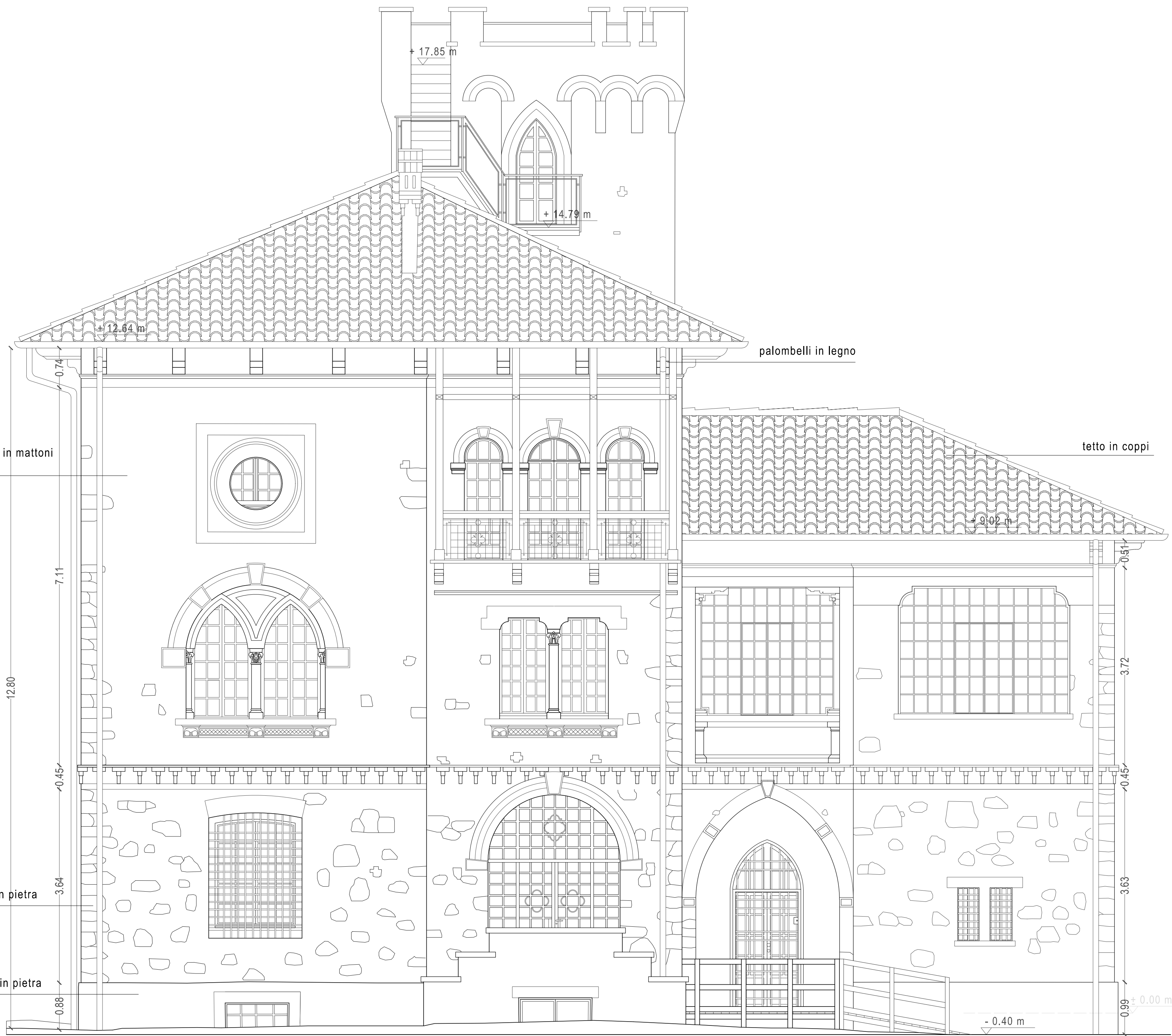
Prospetto OVEST
