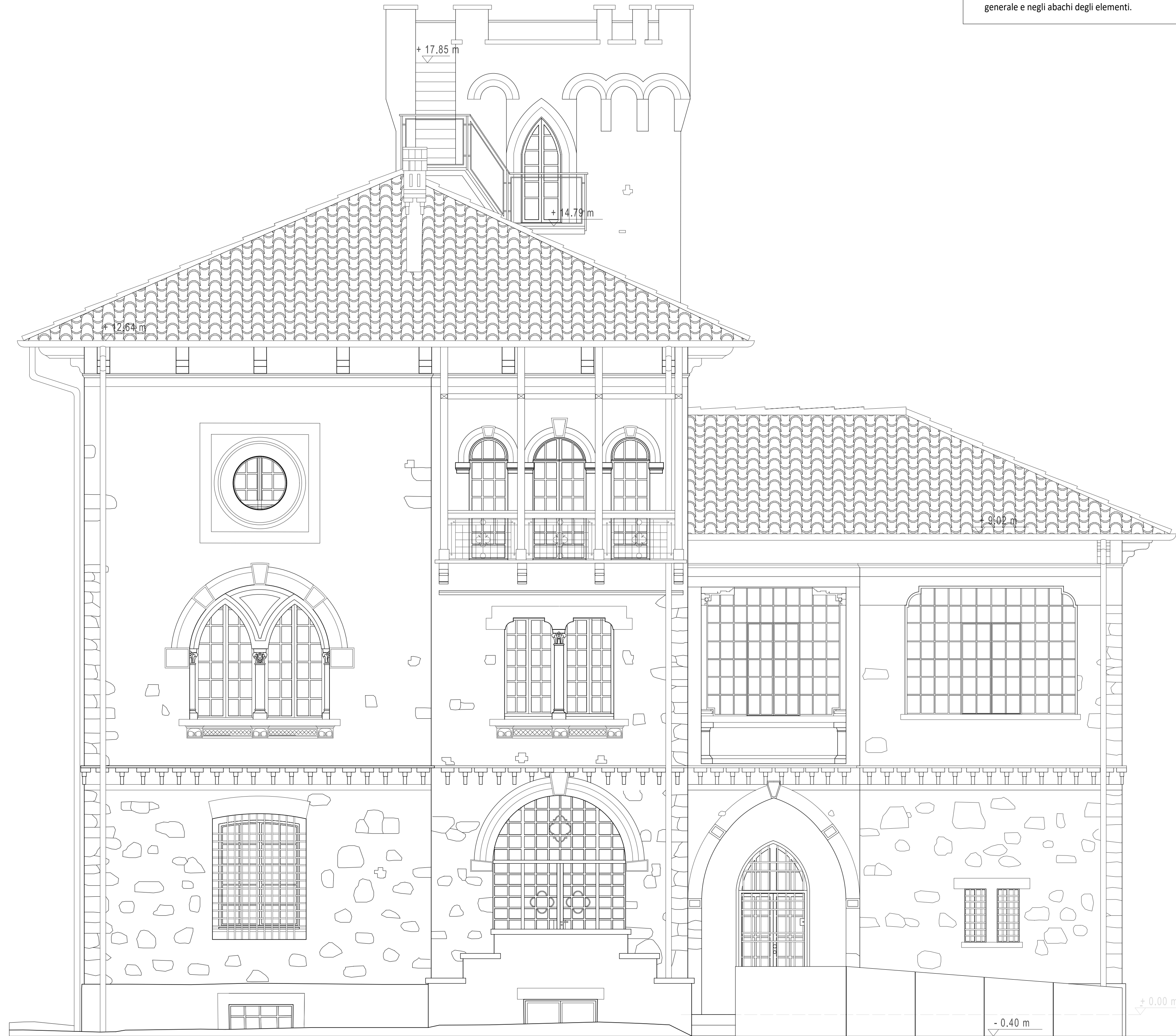
Prospetto OVEST
