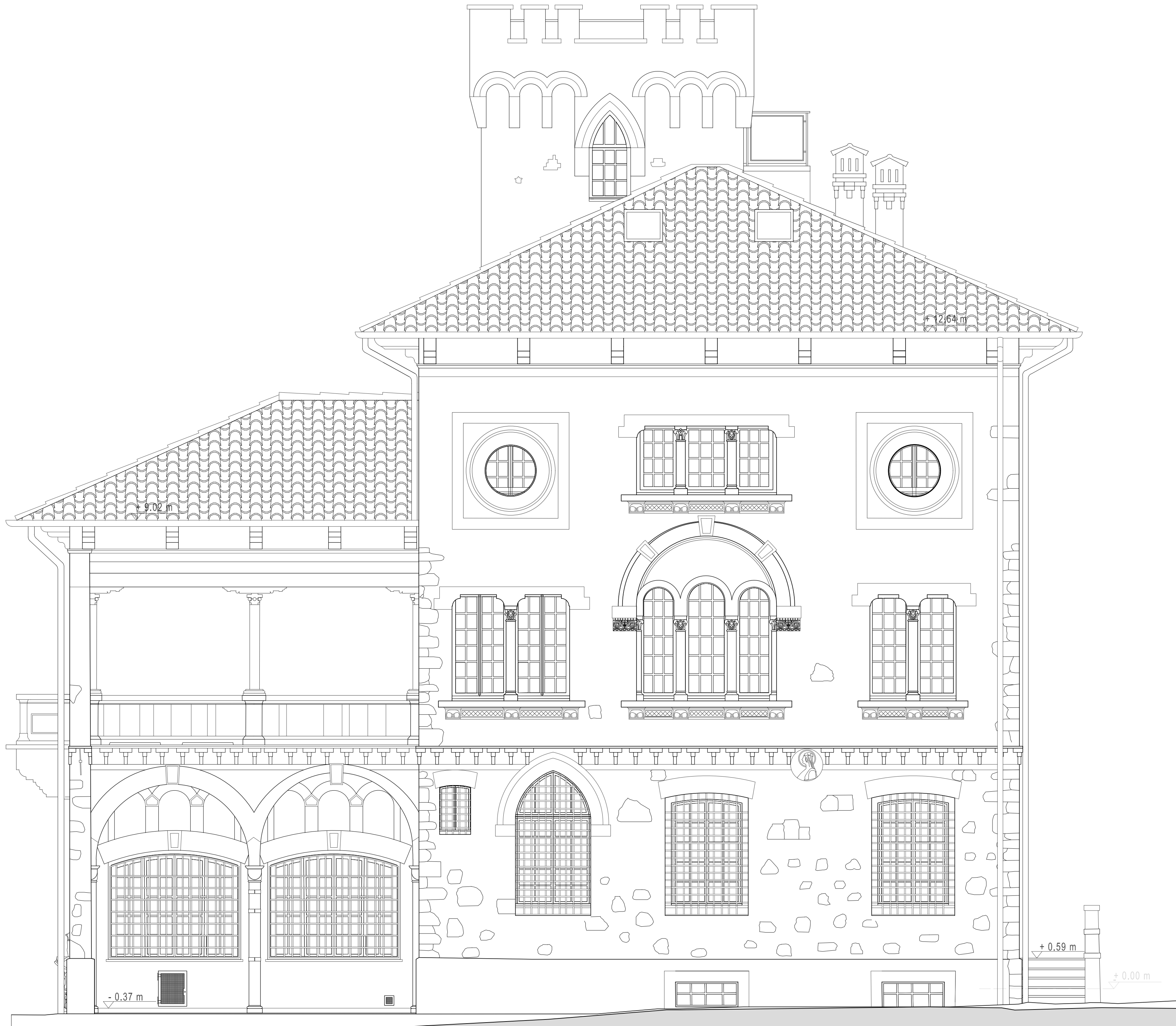
Prospetto NORD
