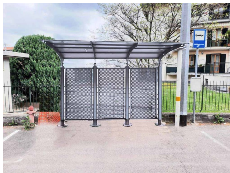
NUOVA PENSILINA A SBALZO dim 300x230x170
