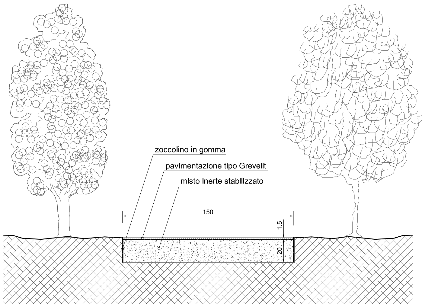
SEZIONE A-A
