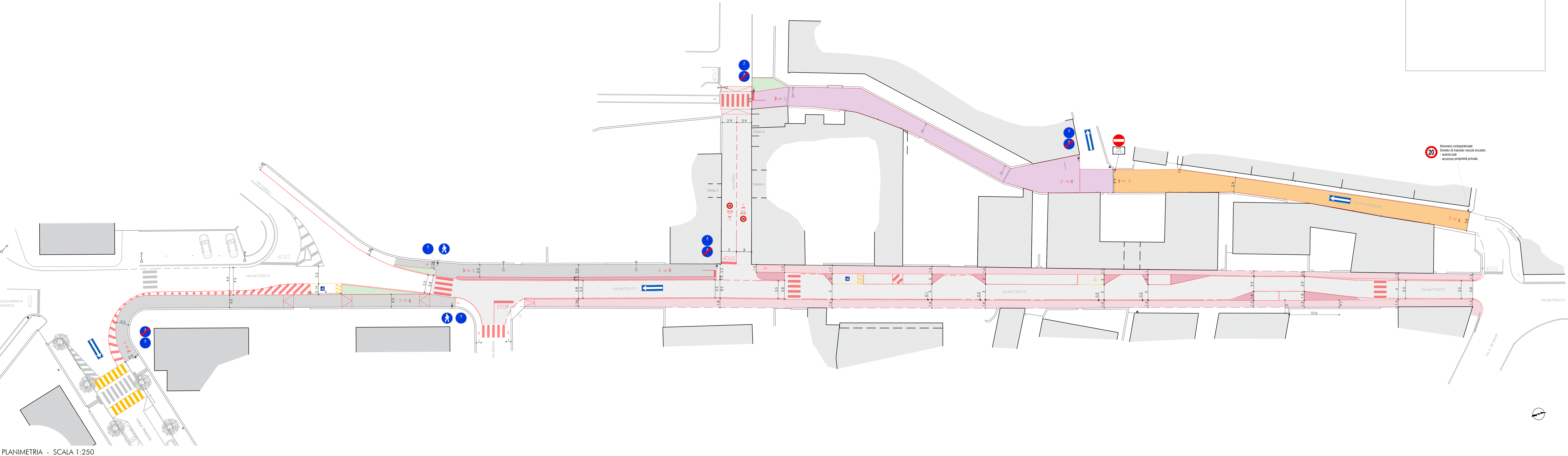
PLANIMETRIA - SCALA 1:250
