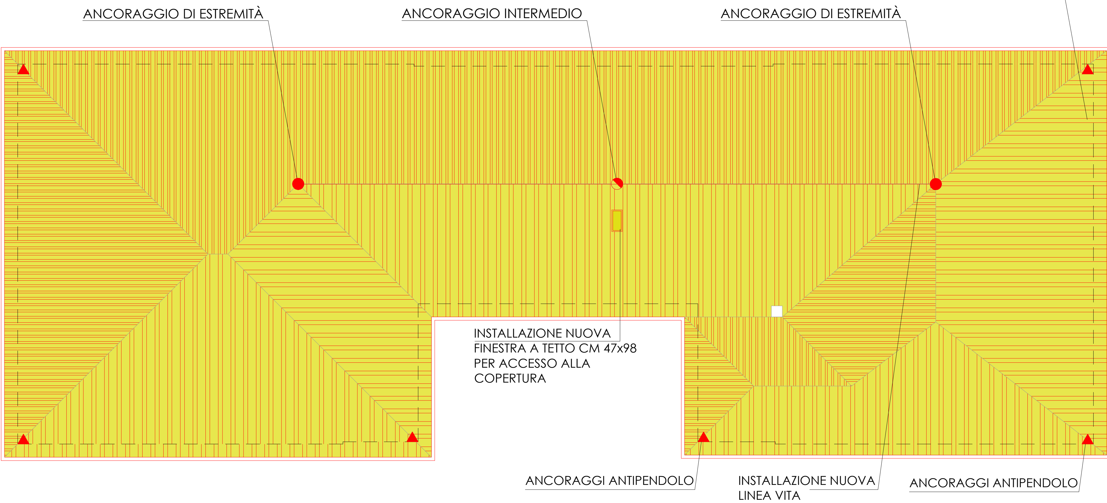
CONFRONTO scala 1:100
