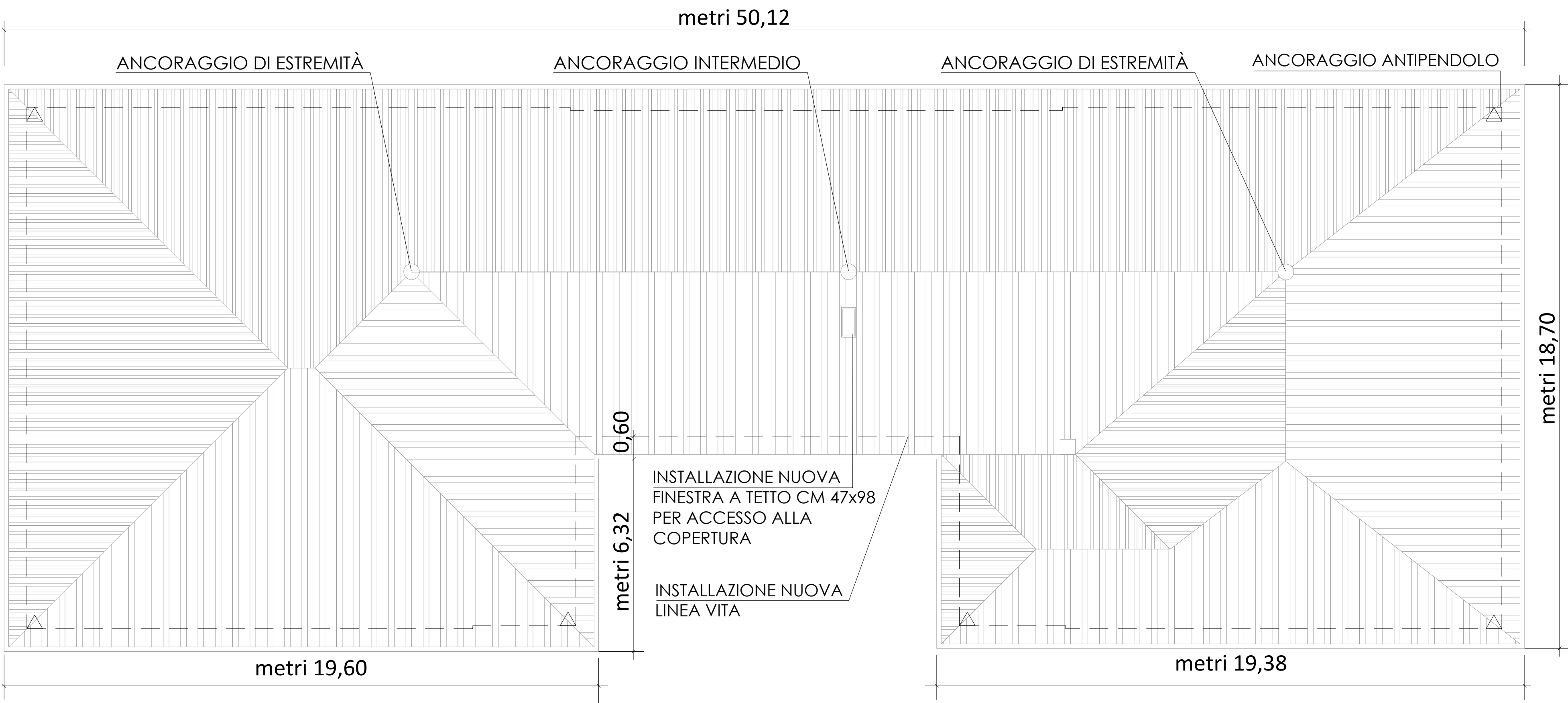
PROGETTO scala 1:100
