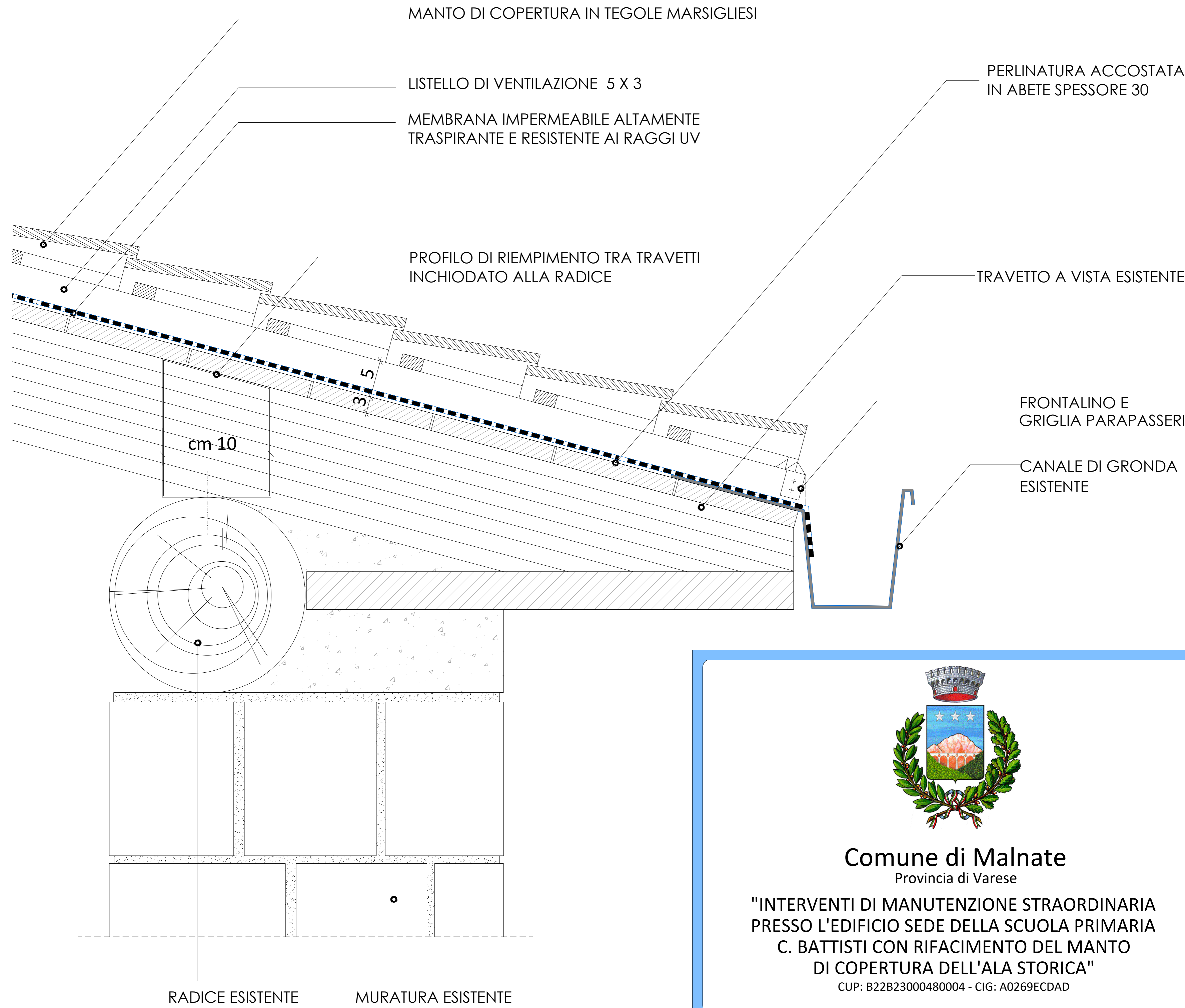
PARTICOLARE DELLA COPERTURA IN PROGETTO
