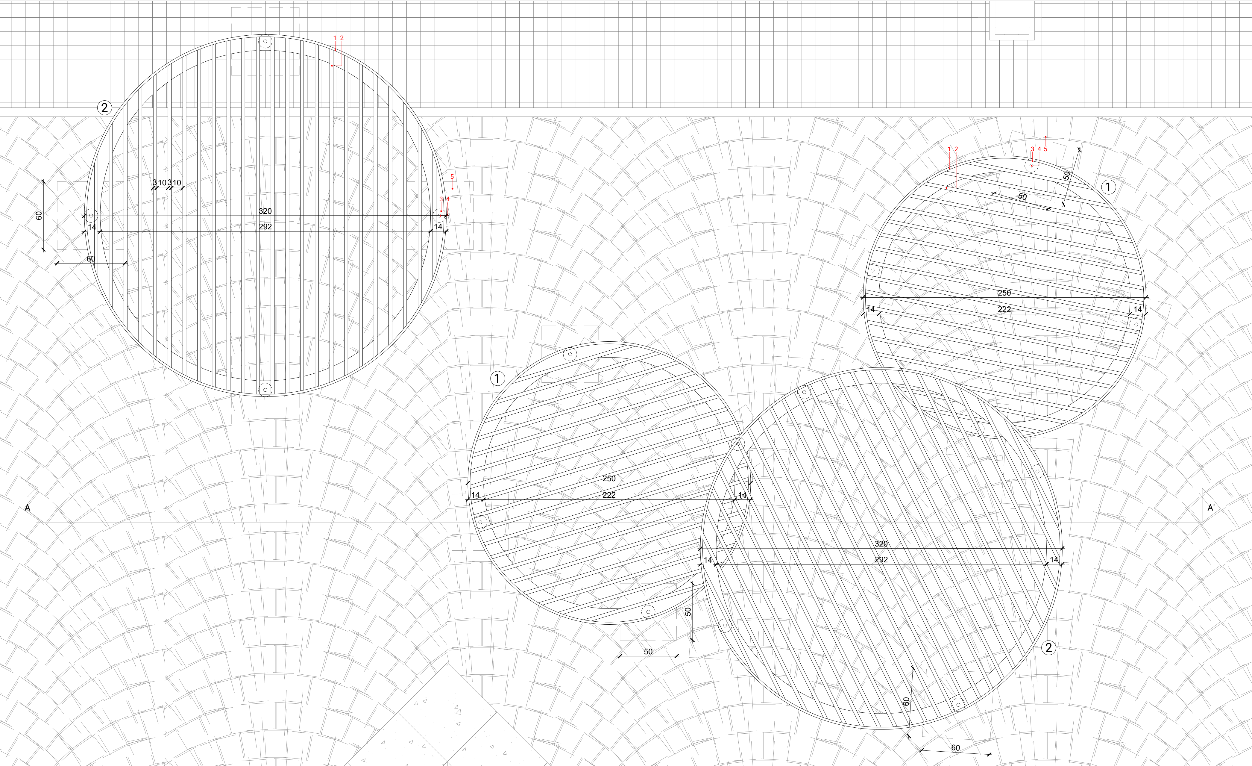
DETTAGLIO A2 - Estratto planimetrico
