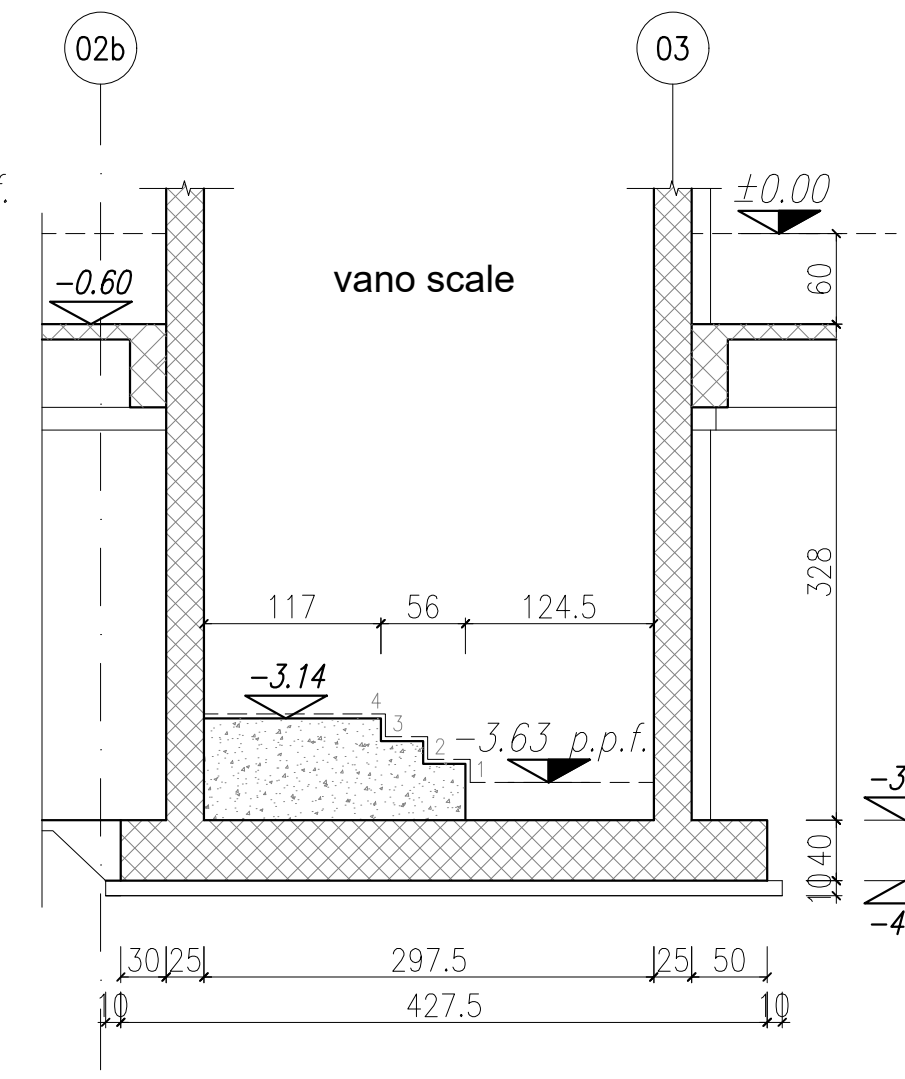
Sezione 1-1 scala 1:50
