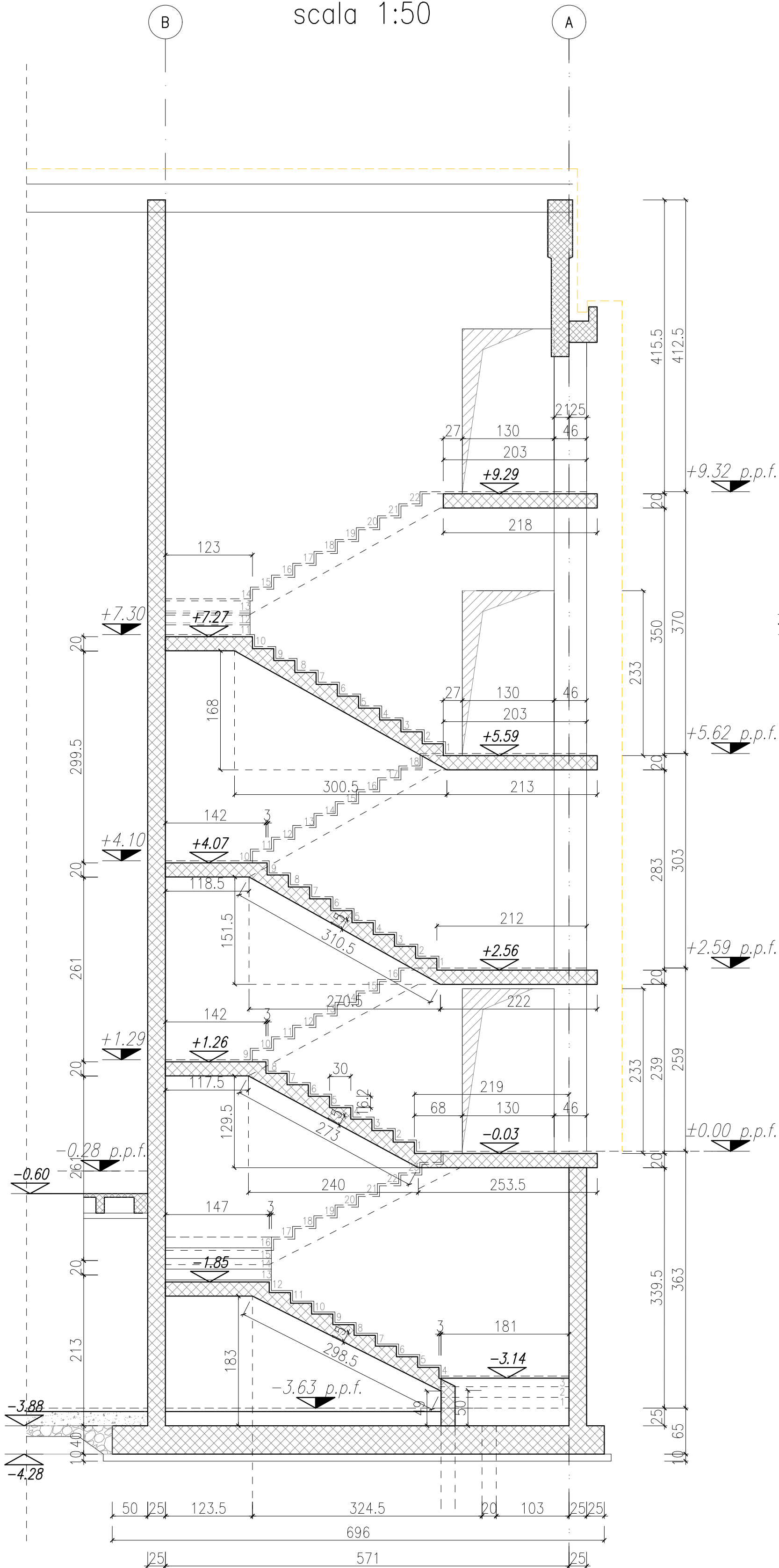
Sezione 2-2 scala 1:50
