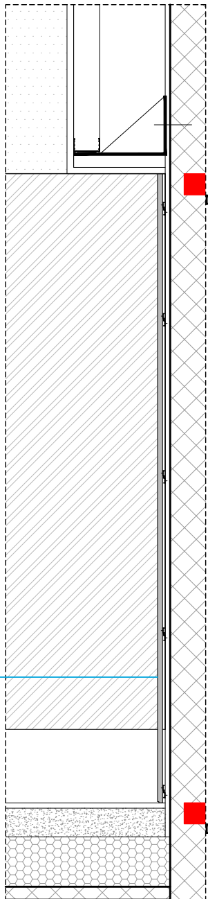
STRALCIO SEZIONE scala 1:20
