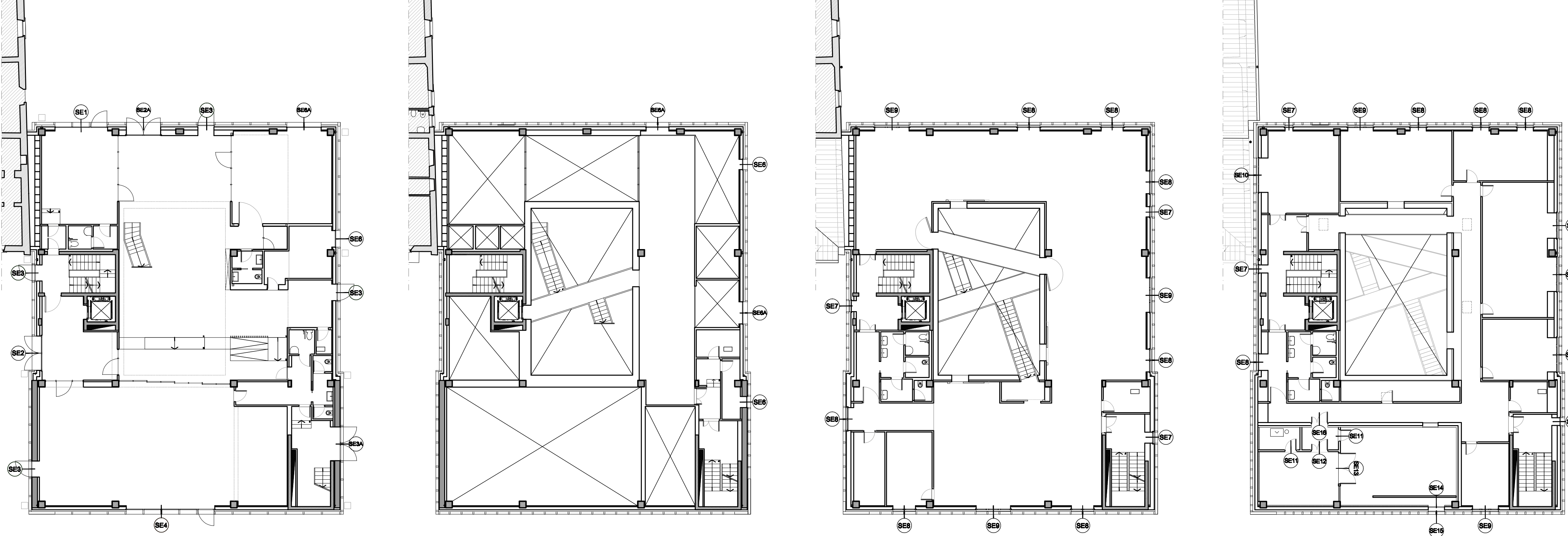
PIANO TERRA PIANO RIALZATO PIANO PRIMO PIANO SECONDO
