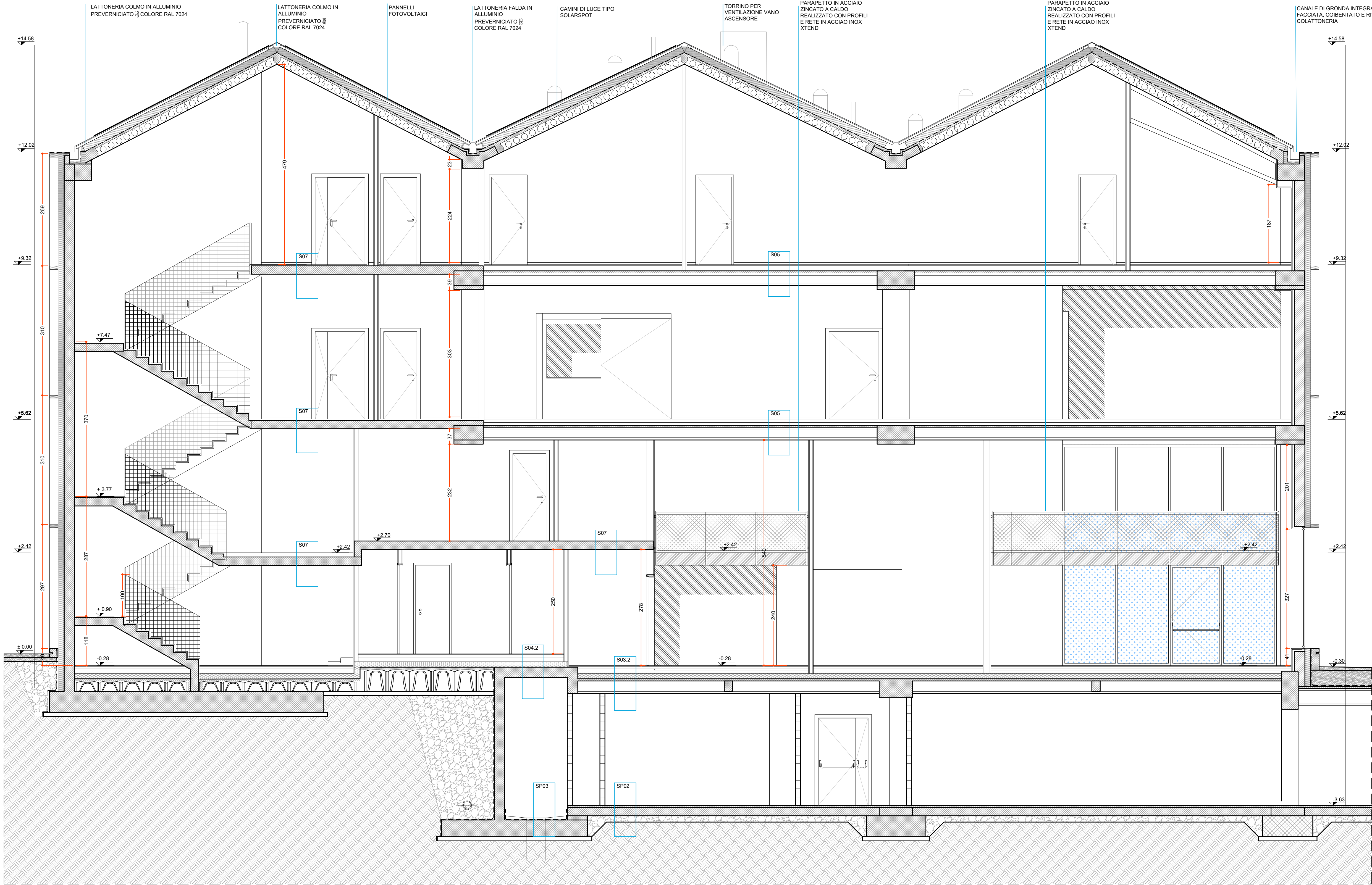
SEZIONE AA'
