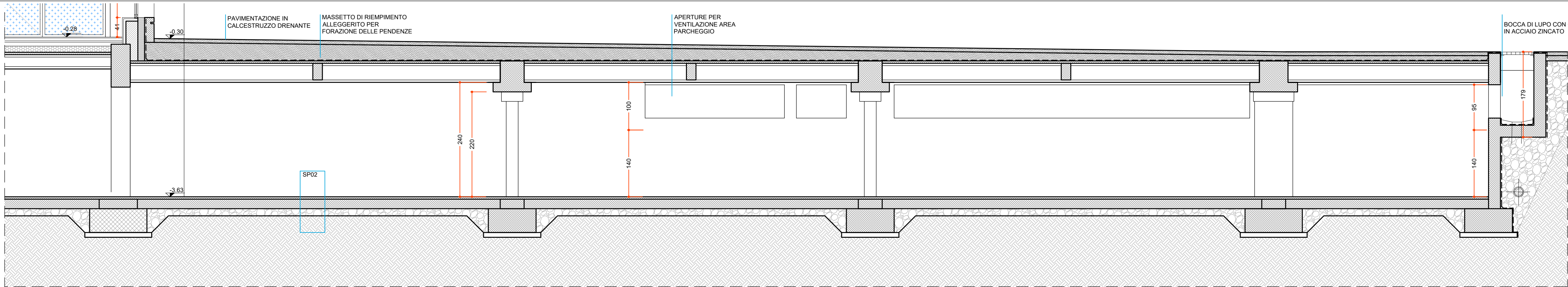
SEZIONE AA' - PARCHEGGIO INTERRATO
