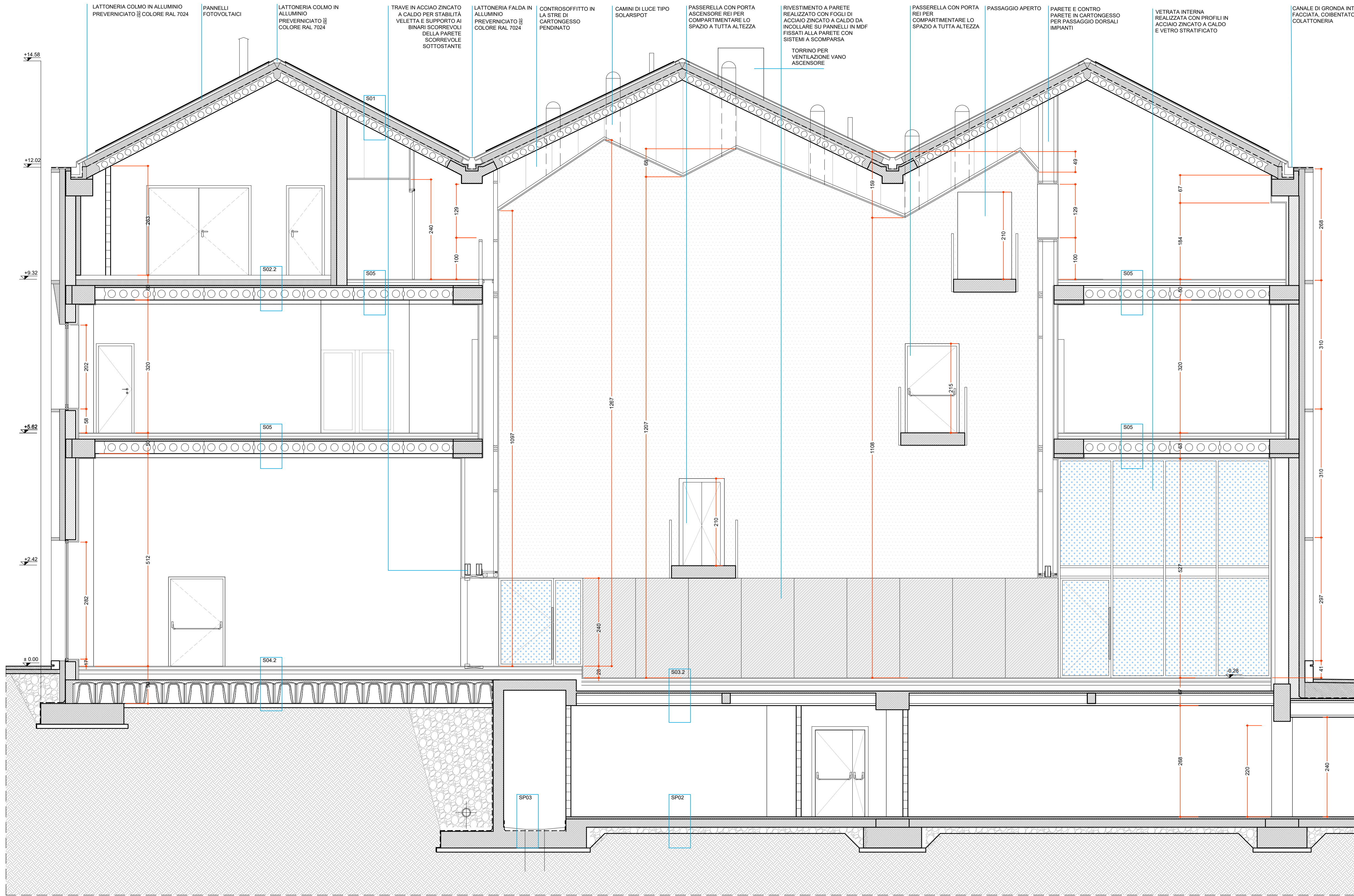
SEZIONE BB'
