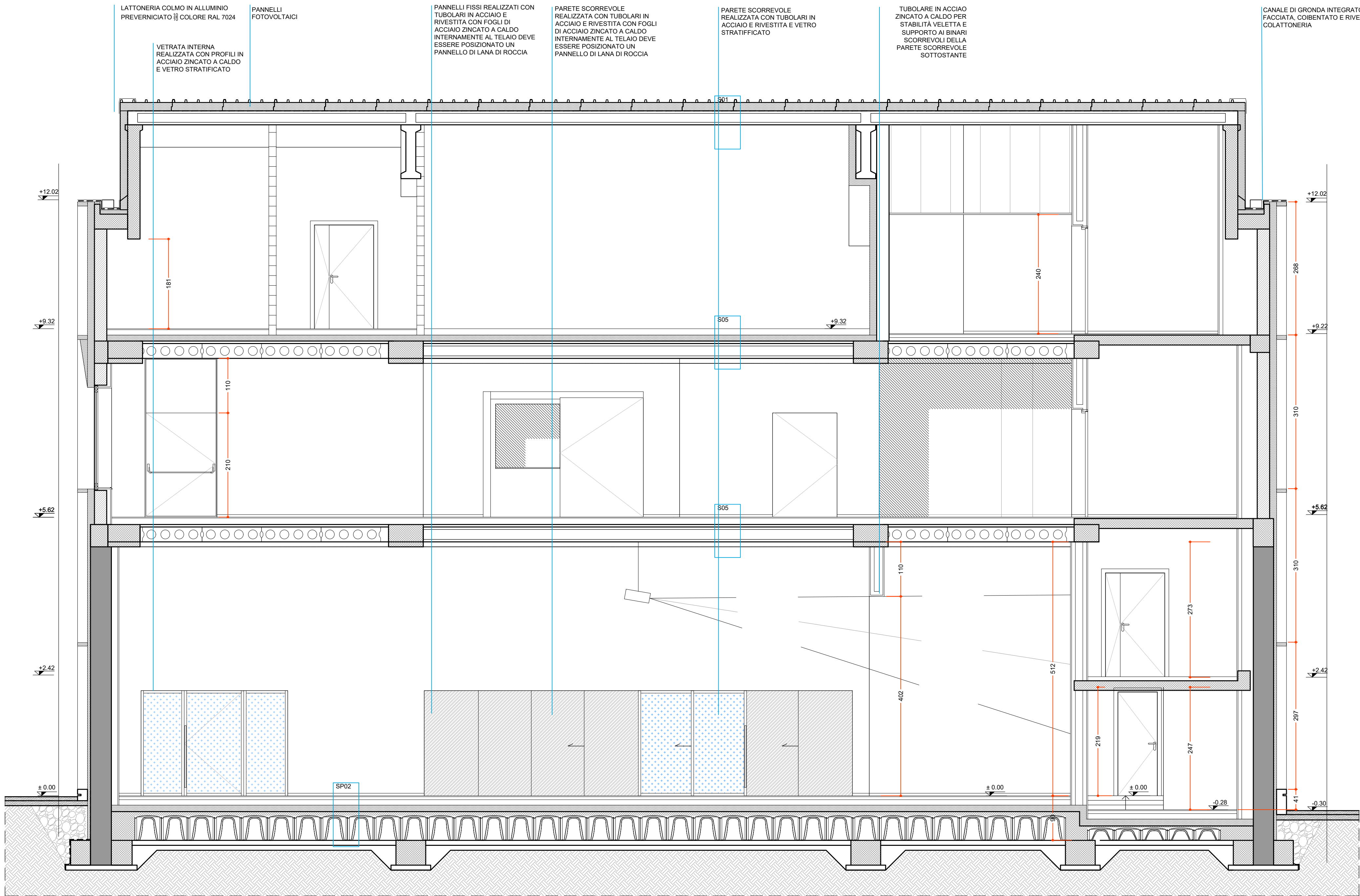
SEZIONE CC'
