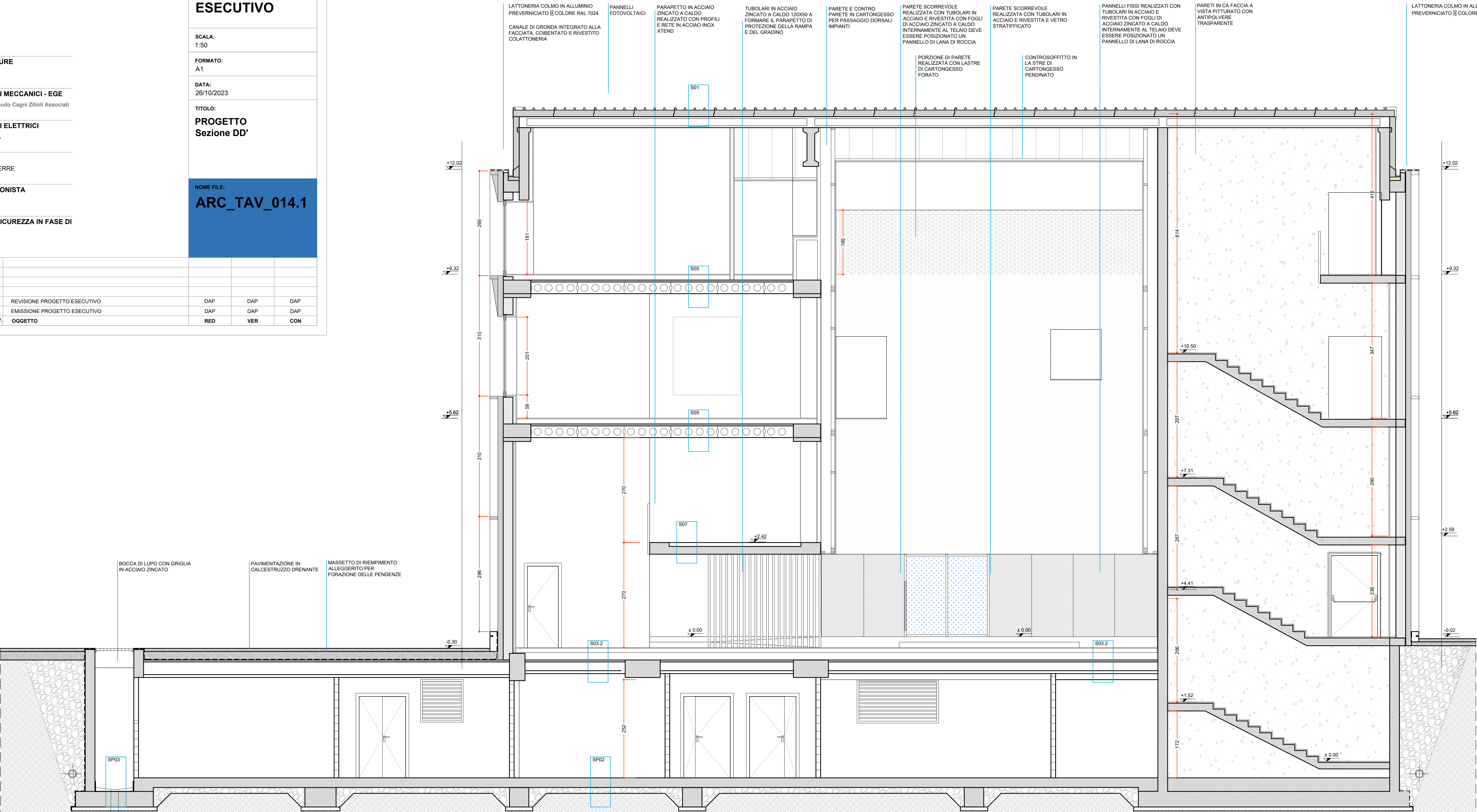
SEZIONE DD'
