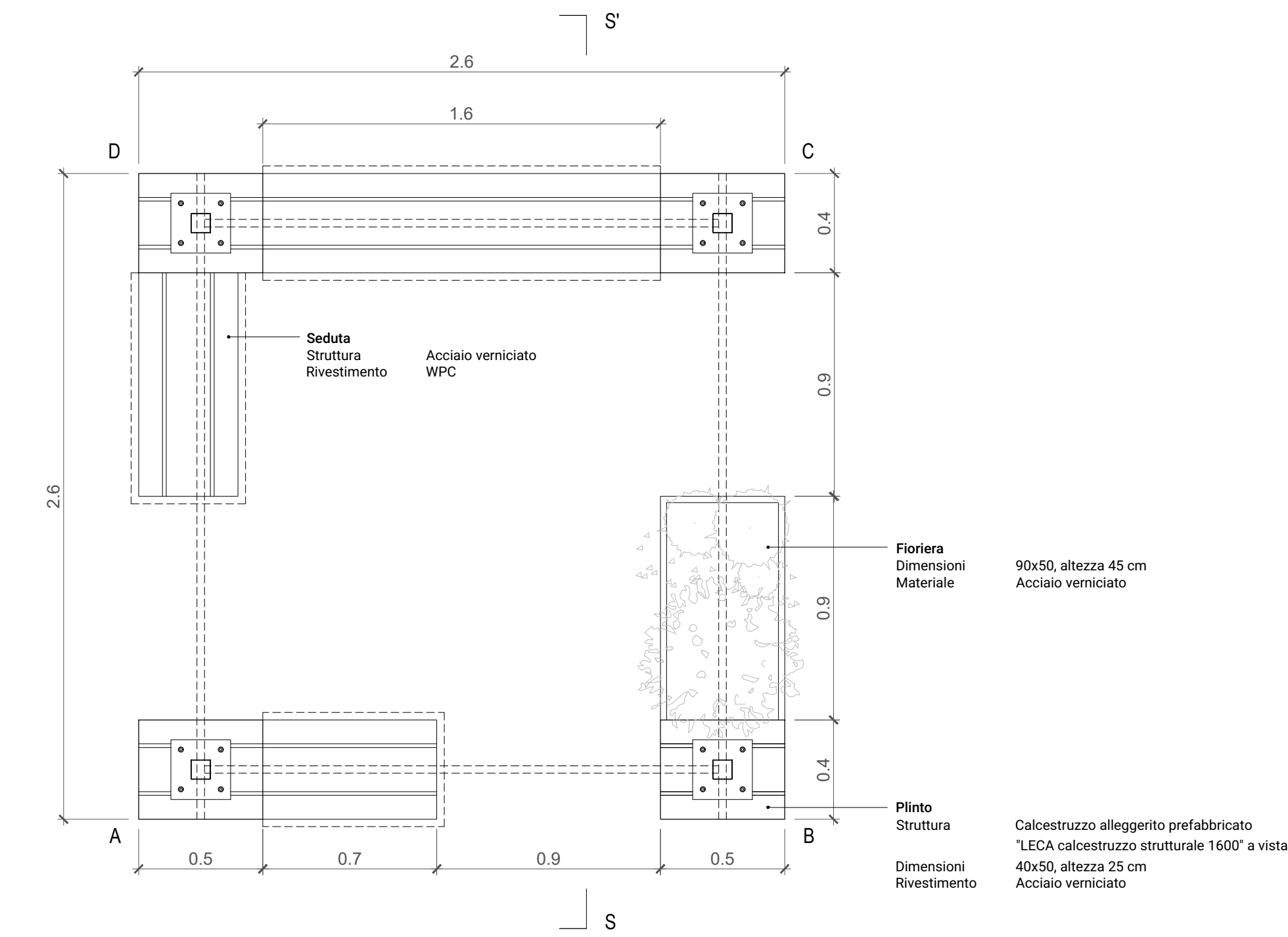
Pianta
