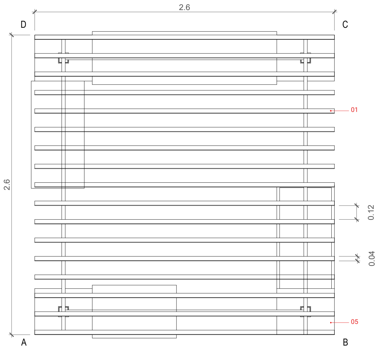
Pianta della copertura
