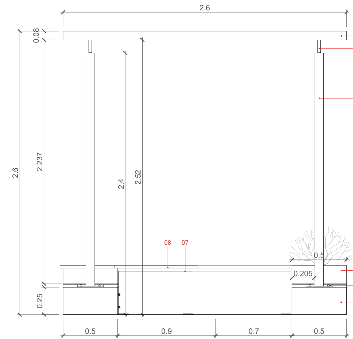
Prospetto AB
