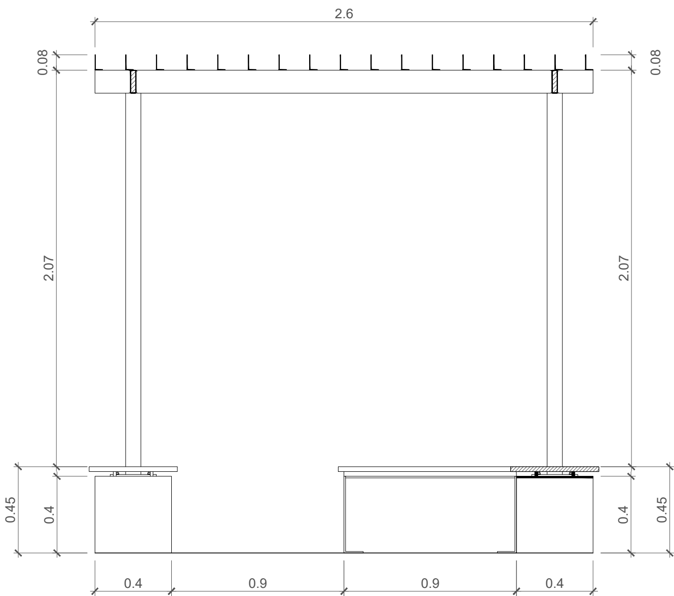
Sezione SS'
