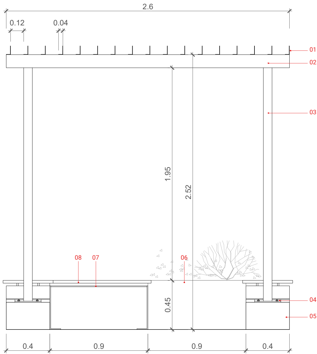
Prospetto DA
