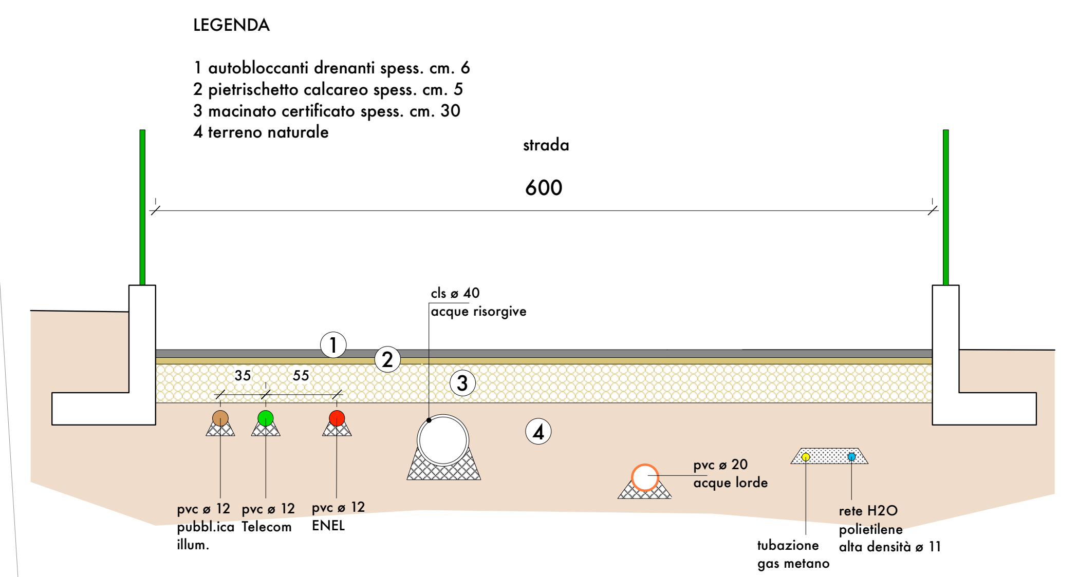
sezione 1-1 scala 1 : 30
